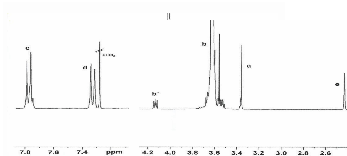
Figura 1. Espectro 1 H-RMN del polietilenglicol tosulado en cloroformo deuterado a 25°C (ver la asignación de señales en el esquema 1).
