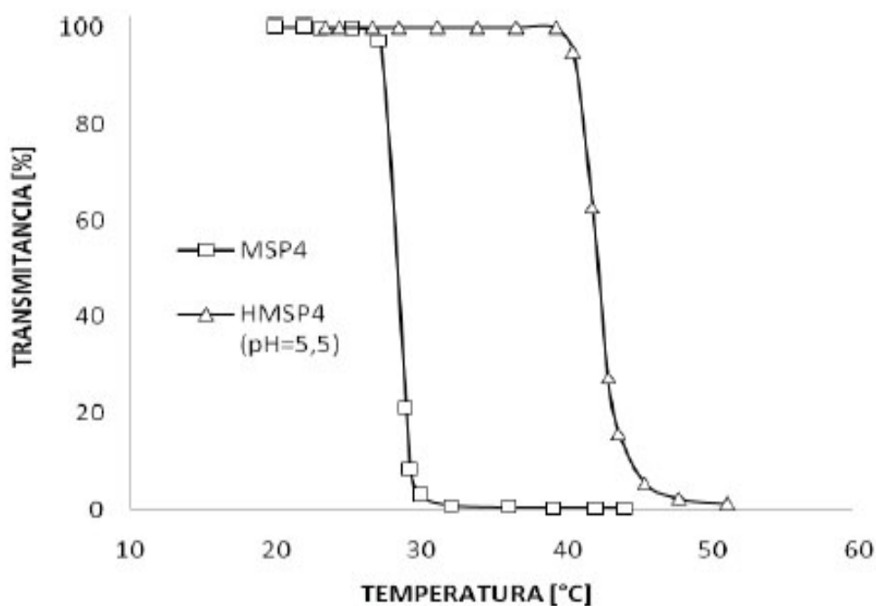
Figura 4. Determinación de LCST para la muestra MSP4 antes (LCST=28°C) y después de la hidrólisis (H-MSP4, pH 5,5, LCST=42°C).
