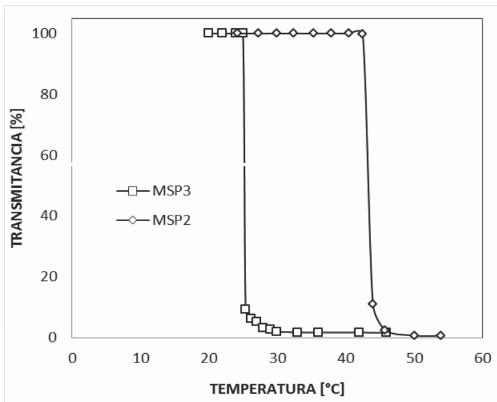
Figura 3. Determinación de LCST para la muestras MSP2 (LCST=42°C) y MSP3 (LCST=24°C).
