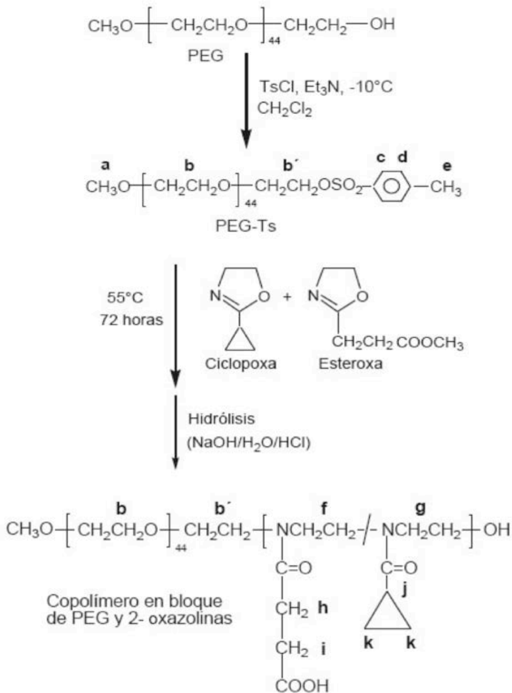
Esquema 1. Tosilación del PEG y subsecuente polimerización de las 2-oxazolinias mediante el PEG tosilado.
