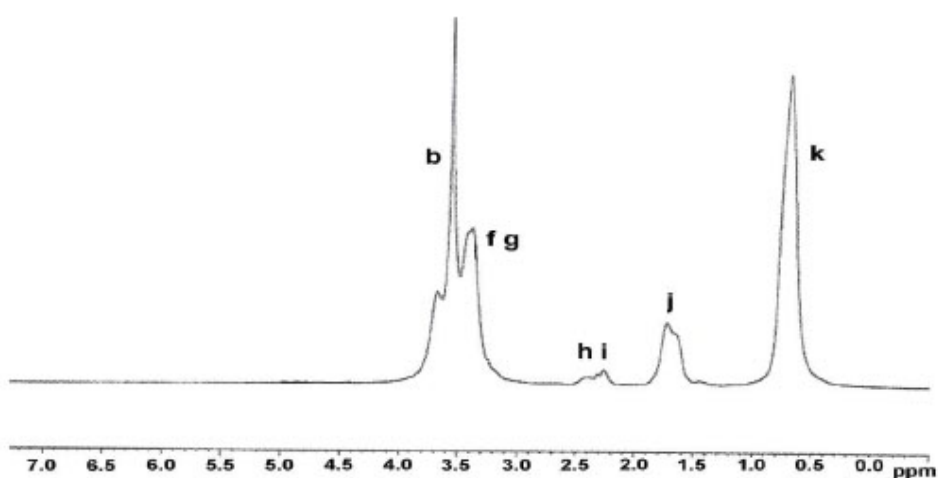
Figura 2. Espectro ^1\text{H} -RMN del copolímero hidrolizado H-MSP4 en agua deuterada. La asignación de señales se realizó según el esquema 1.
