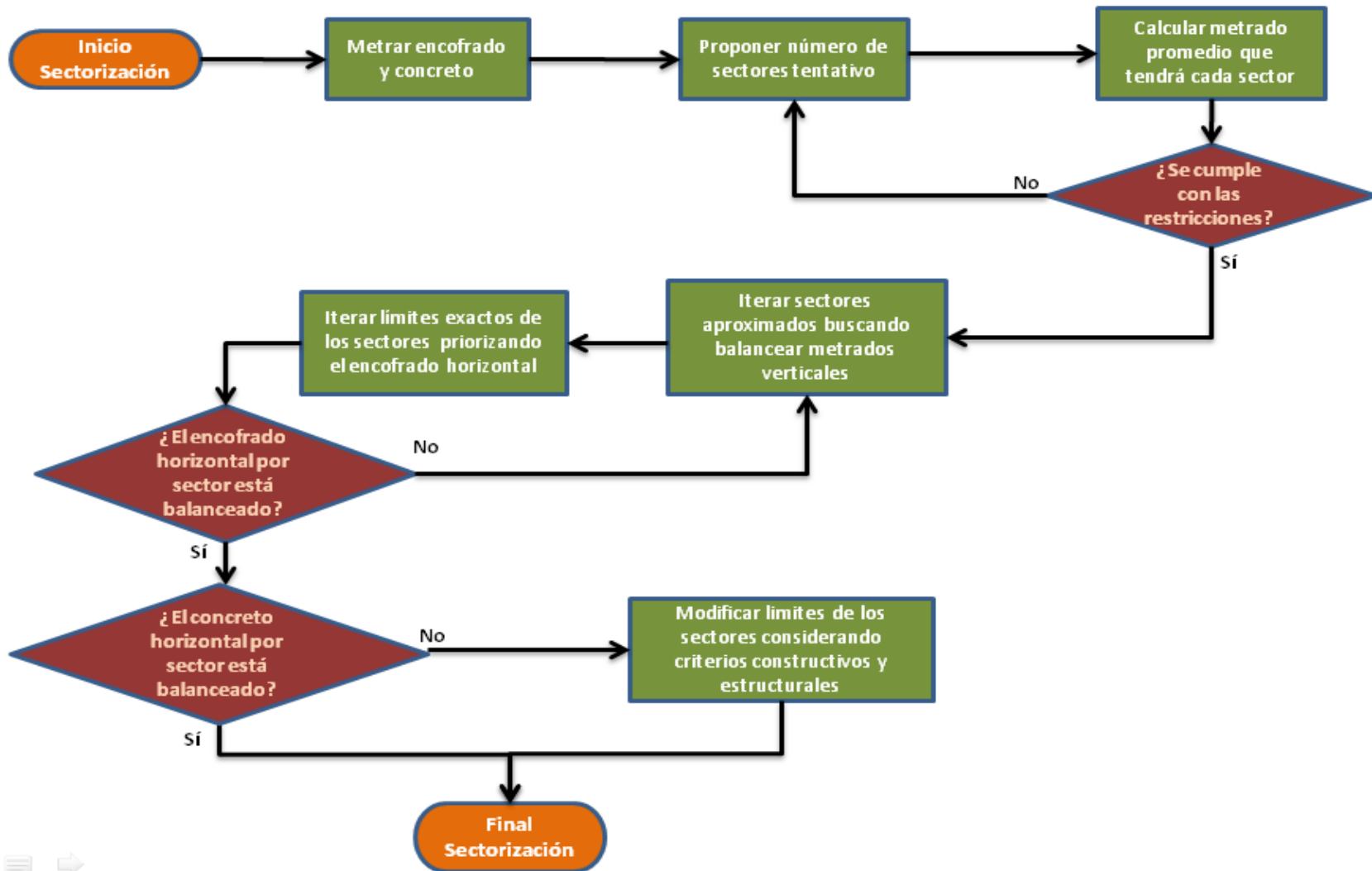
Flujo de procedimiento de sectorización (Fuente: Edifica)
