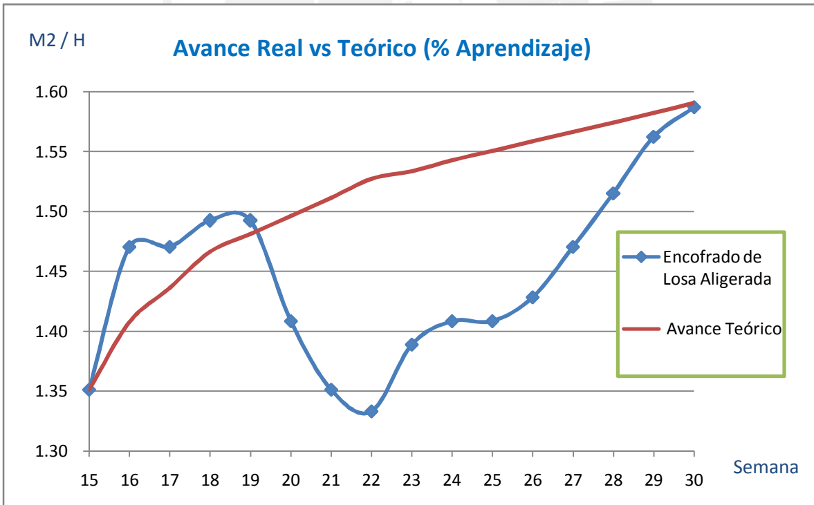
Grafico de avance diario de la partida encofrado de losa aligerada (Fuente Propia)
