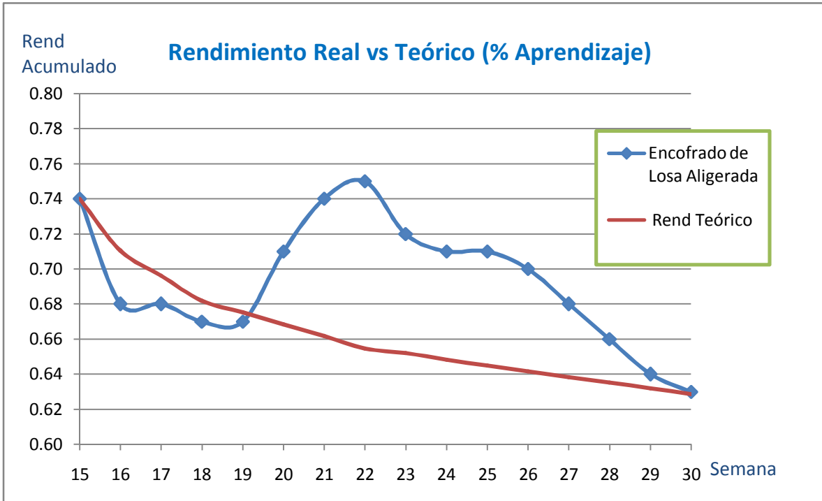
Grafico de Rendimientos Acumulados de la partida encofrado de losa aligerada (Fuente Propia)
