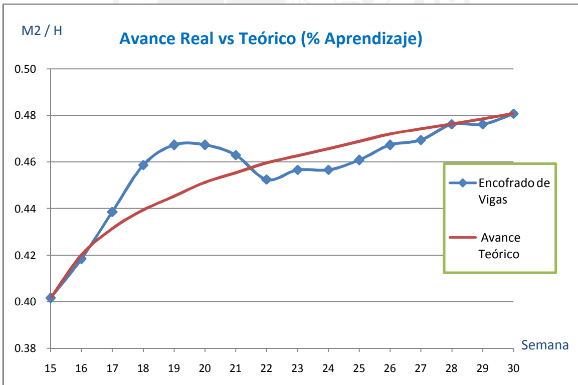
Grafico de avance diario de la partida encofrado de Vigas (Fuente Propia)
