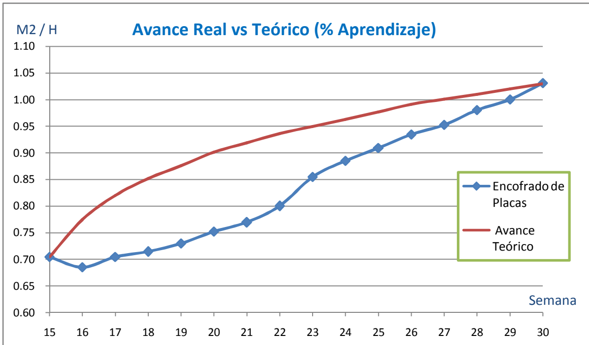
Gráfico de avance diario de la partida encofrado de placas (Fuente Propia)
