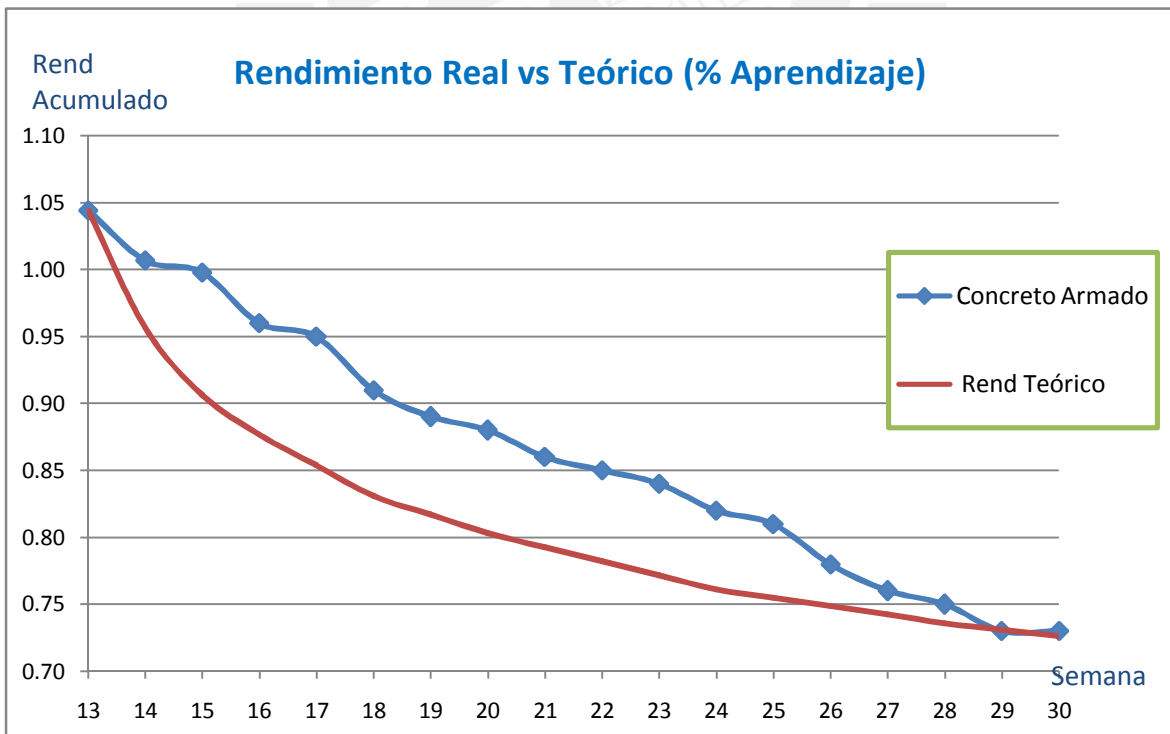
Grafico de Rendimientos Acumulados de la partida Concreto Armado (Fuente Propia)
