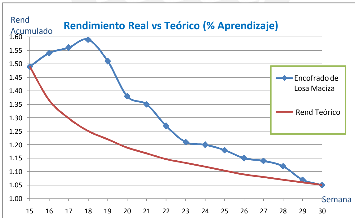
Grafico de Rendimientos Acumulados de la partida encofrado de losa Maciza (Fuente Propia)
