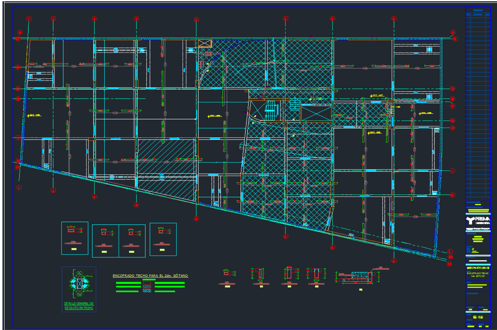
Plano de Encofrado sótanos Proyecto Barranco 360 (Fuente: Edifica)
