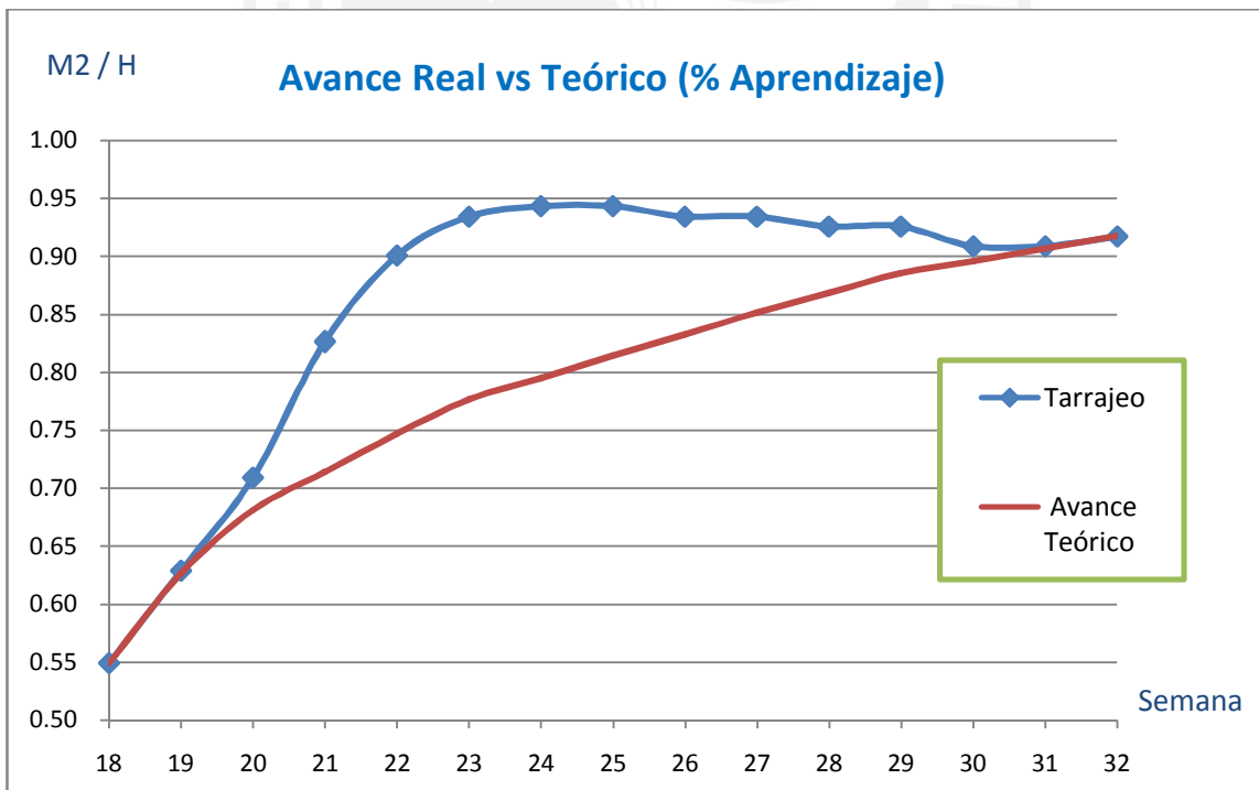
Gráfico de avance diario de la partida Tarrajeo (Fuente Propia)
