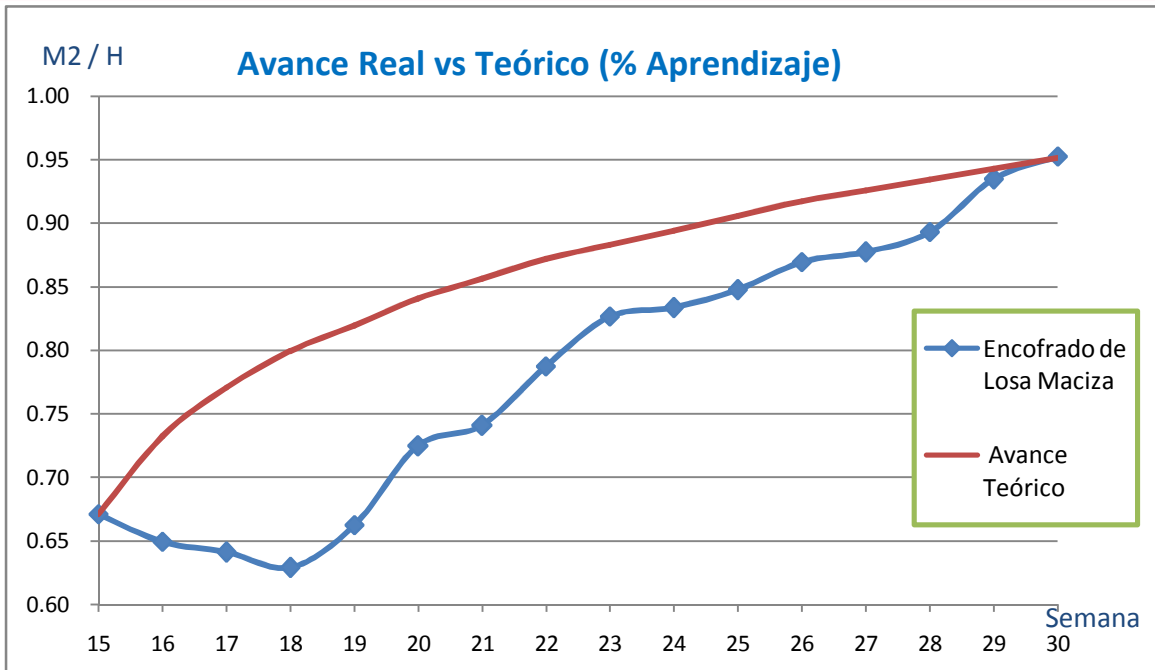
Grafico de avance diario de la partida encofrado de losa maciza (Fuente Propia)
