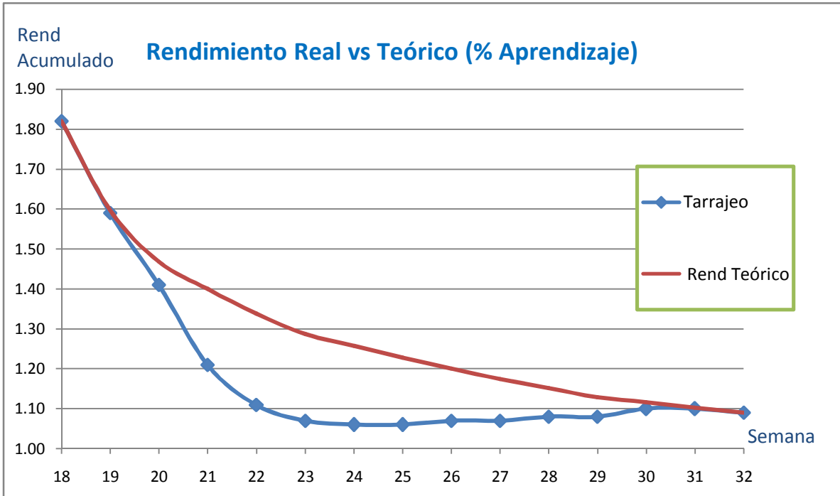
Gráfico de Rendimientos Acumulados de la partida Tarrajeo (Fuente Propia)
