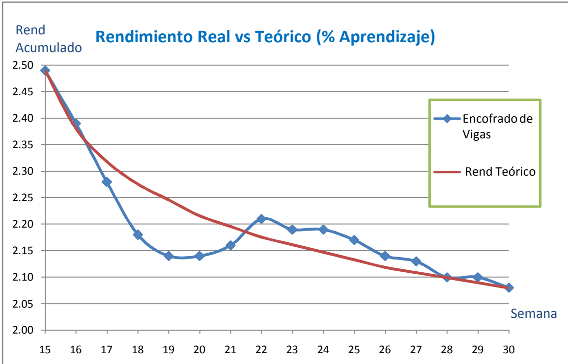
Grafico de Rendimientos Acumulados de la partida encofrado de Vigas (Fuente Propia)
