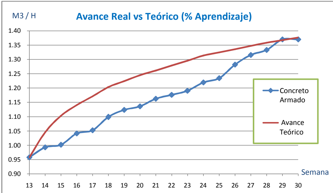
Grafico de avance diario de la partida Concreto Armado (Fuente Propia)
