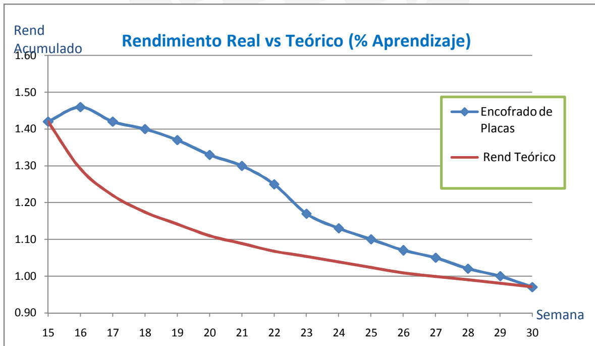
Gráfico de Rendimientos Acumulados de la partida encofrado de placas (Fuente Propia)
