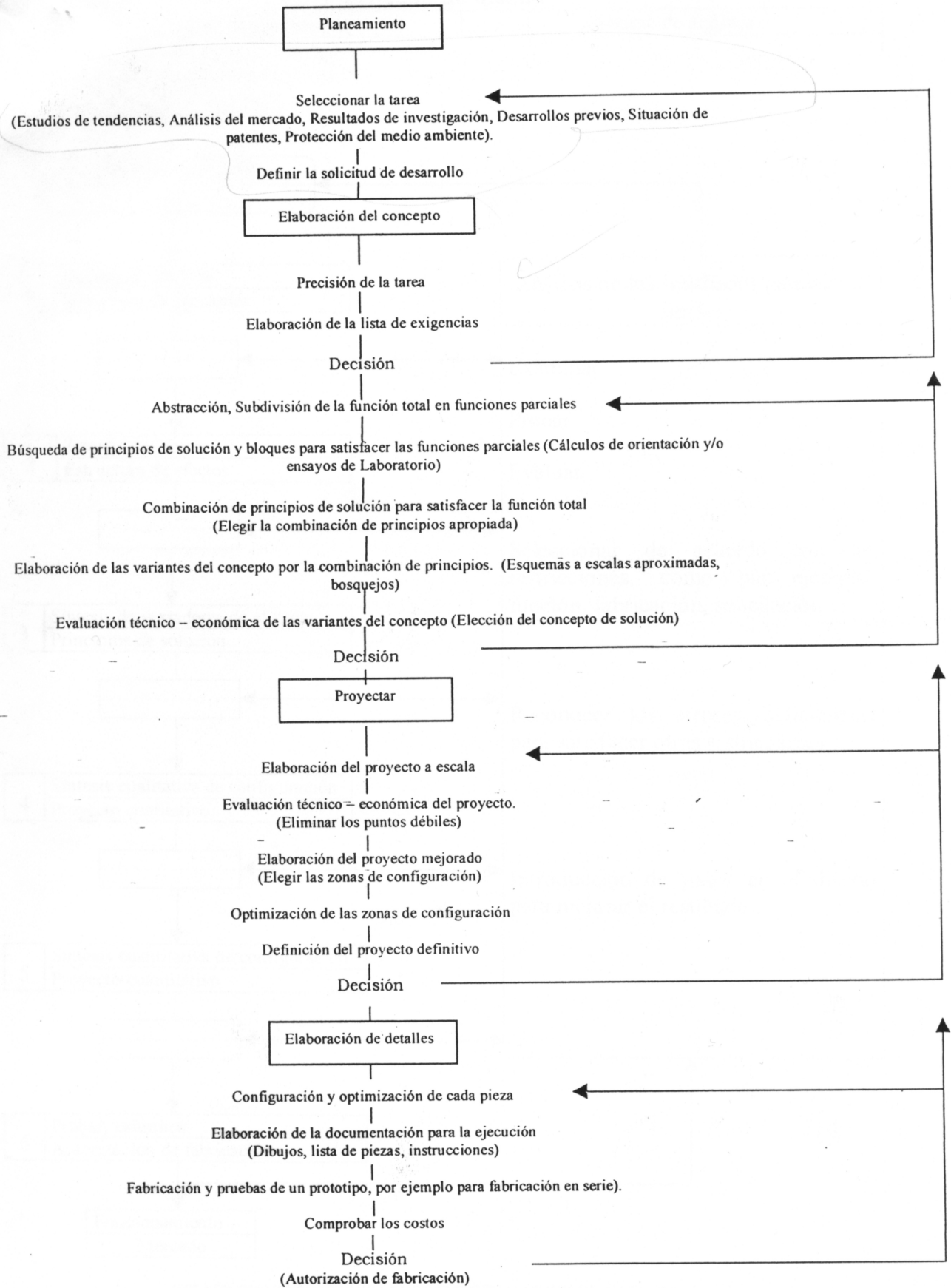
VDI 2222 HOJA 1 (KONSTRUKTIONSMETHODIK, KONZIPHEREN TECHNISCHER PRODUKTE, 1973) Fig. 1.01. Plan de Trabajo para obtener nuevos productos
