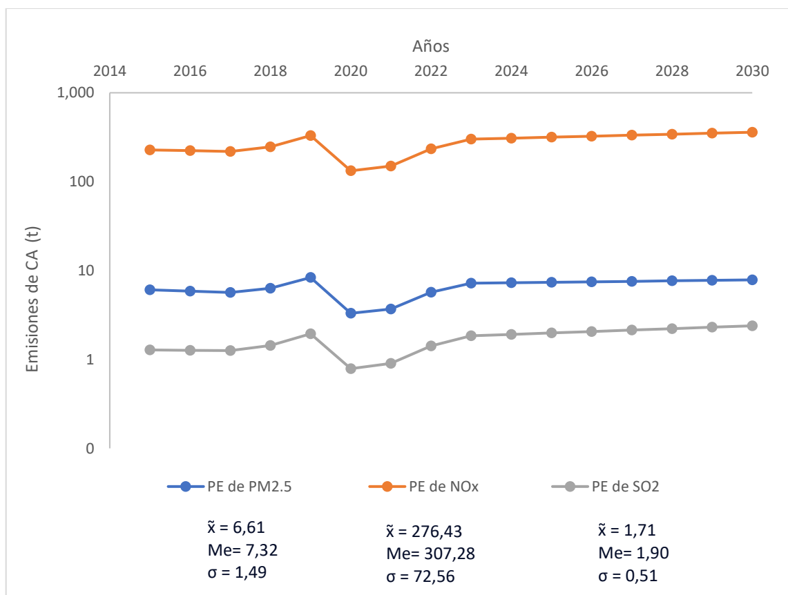
Figura 10: Emisiones de CA ( PM_{2,5} , NO_x y SO_2 ) de la Línea 1 (PE)
