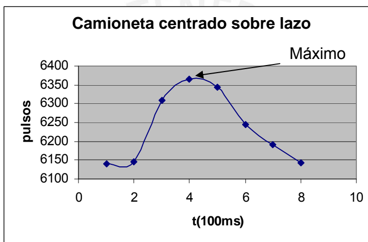
Figura 4.7: camioneta sobre el lazo inductivo (Ver figura 3.4).
