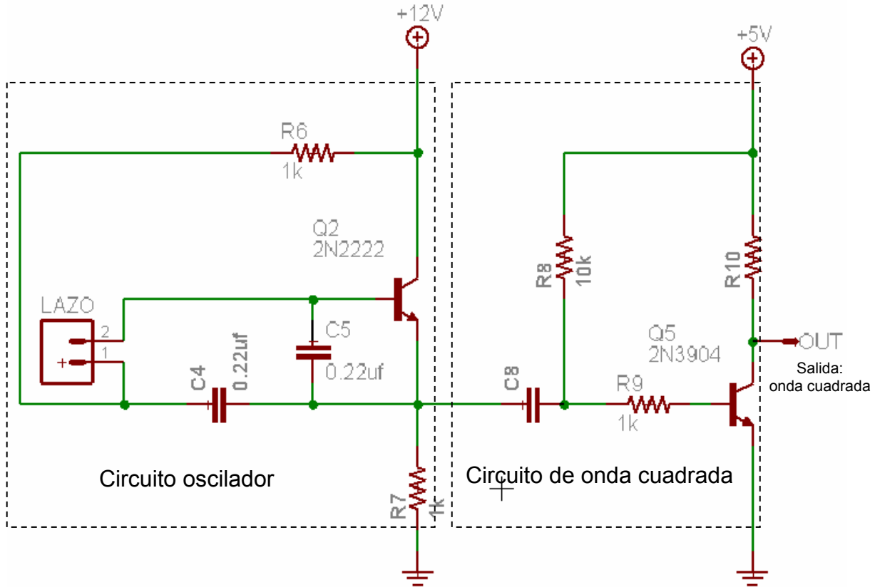
Figura 3.5.1: Circuito esquemático del oscilador y circuito de onda cuadrada
