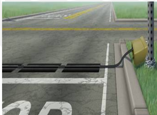
Figura 4.26: Manguera para aforos recubierta con “tapecoat”.
