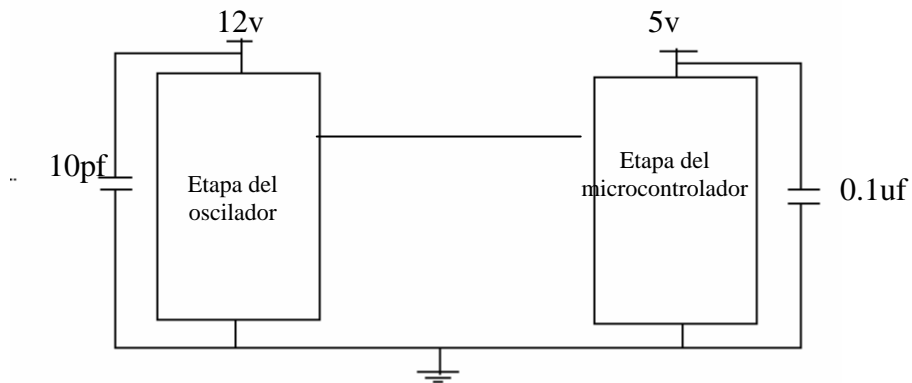
Figura 4.13: Etapas del circuito con dos condensadores
