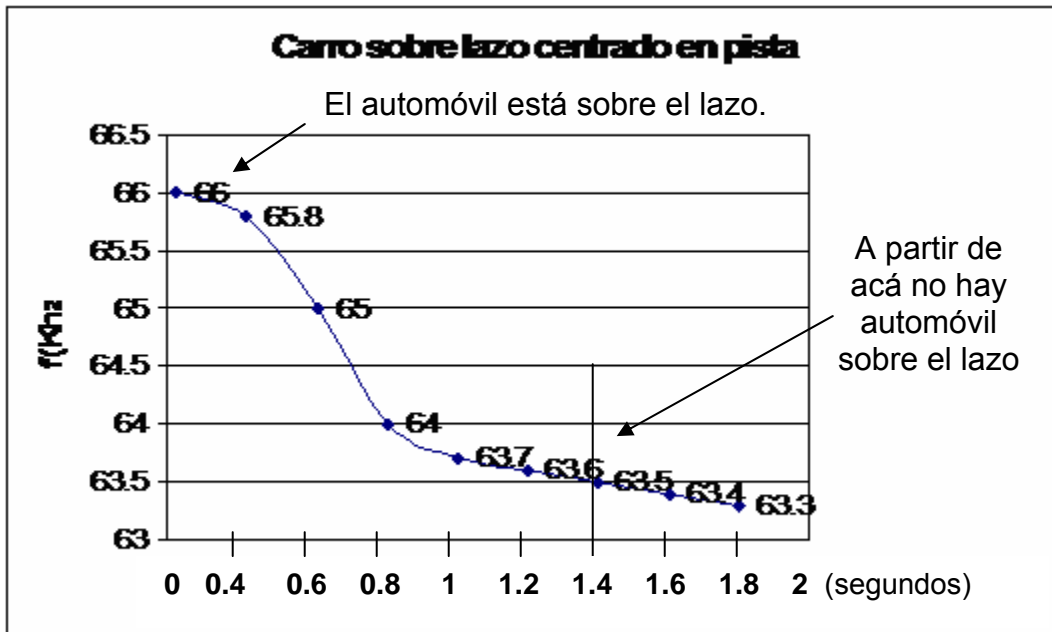
Figura 4.1: Frecuencia según el paso del automóvil sobre el lazo centrado.
