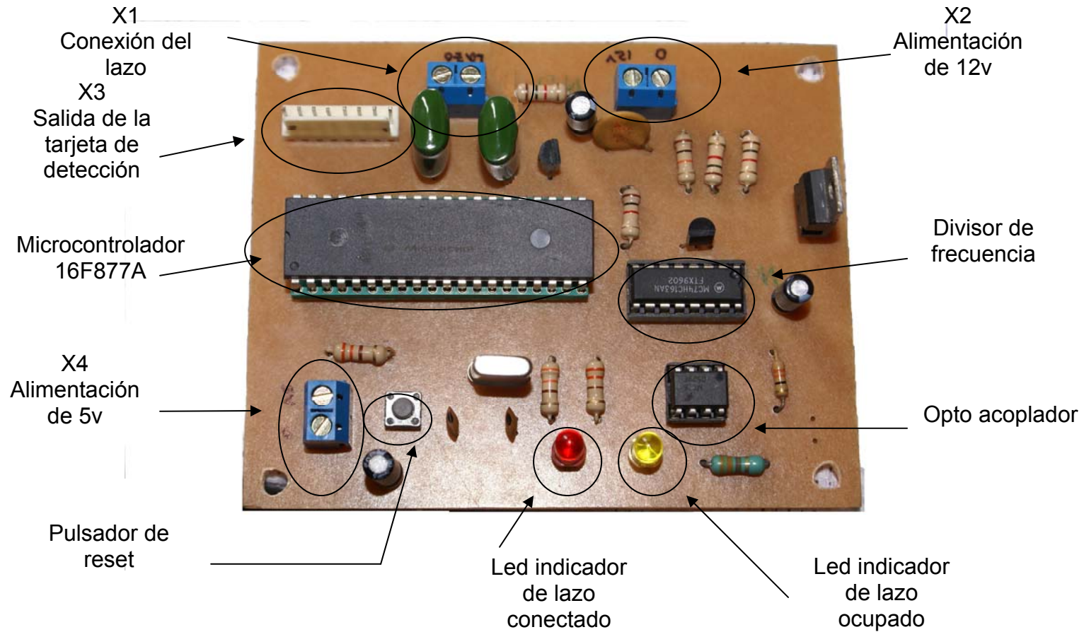
Figura 4.24: Tarjeta del detector de automóviles indicando las borneras de fuente y leds indicadores de funcionamiento.
