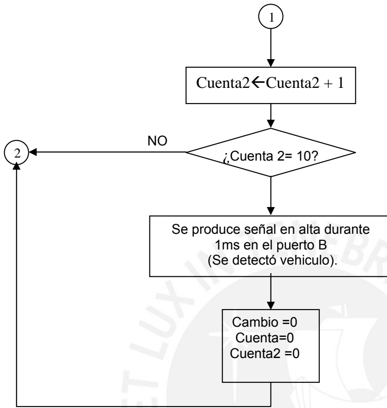
Figura 3.7: Diagrama de flujo del programa de detección.
