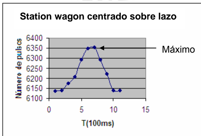
Figura 4.4: Station Wagon pasando sobre lazo inductivo (ver figura 3.4).
