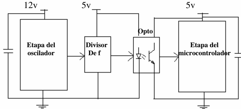
Figura 4.17: Diagrama de bloques del circuito con divisor de frecuencia y opto acoplador.
