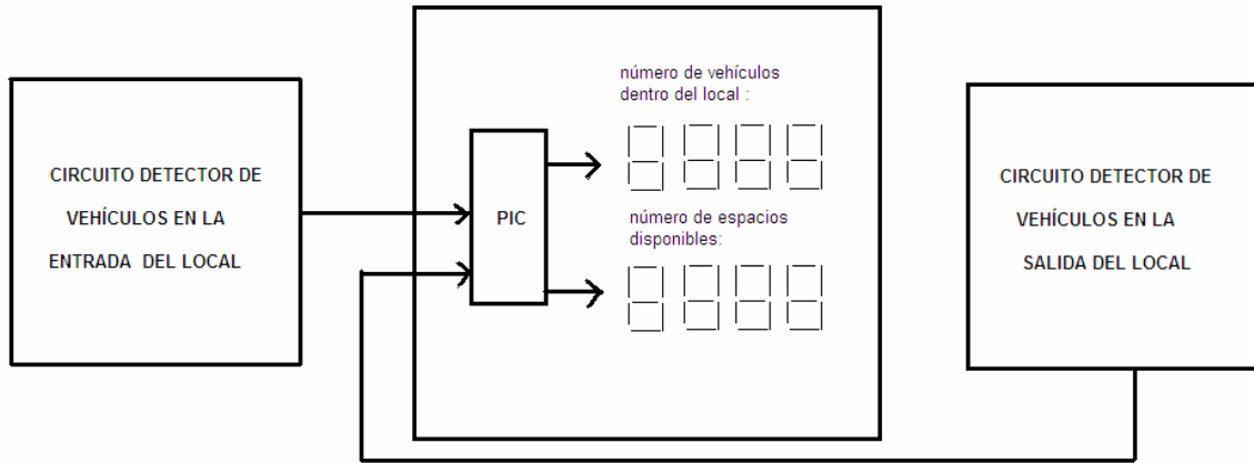
Figura 3.1: Diagrama de bloques del circuito a diseñar.
