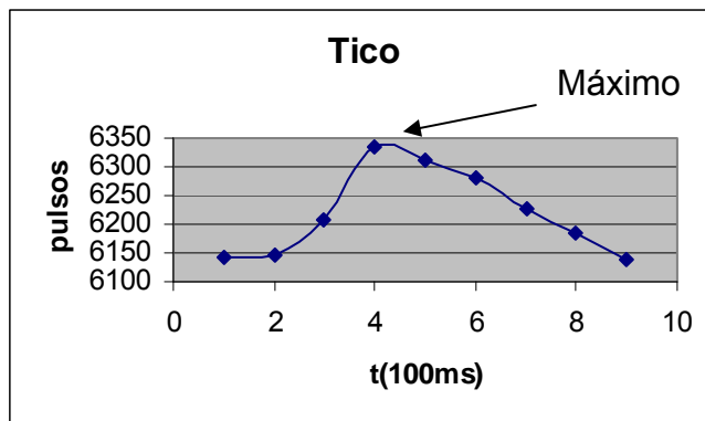
Figura 4.6: Tico pasando sobre el lazo inductivo, (Ver figura 3.4).
