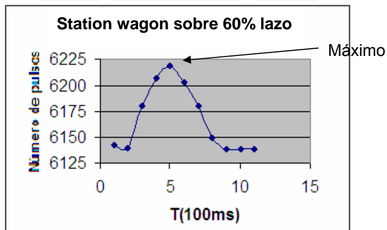
Figura 4.4: Station Wagon pasando sobre lazo inductivo (ver figura 3.4).
