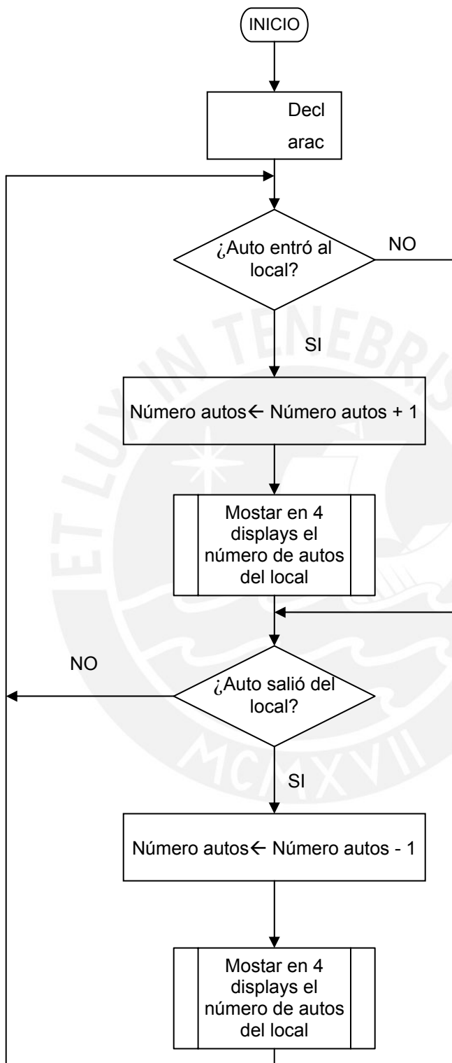
Figura 3.8: Diagrama de flujo del programa principal
