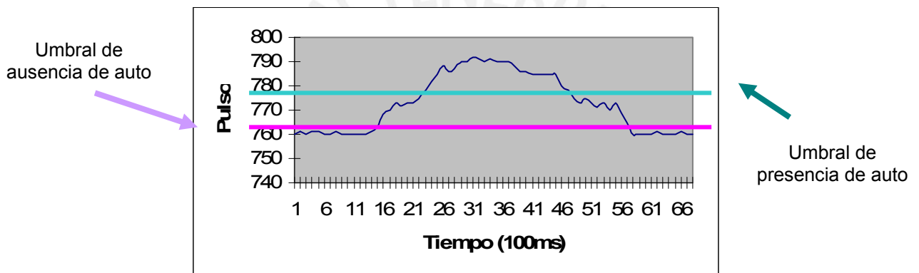
Figura 4.22: Señalización de los umbrales para los dos casos.
