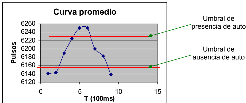
Figura 4.8: Curva promedio del paso de un automóvil sobre el lazo inductor, respecto al número de pulsos cada 100ms.
