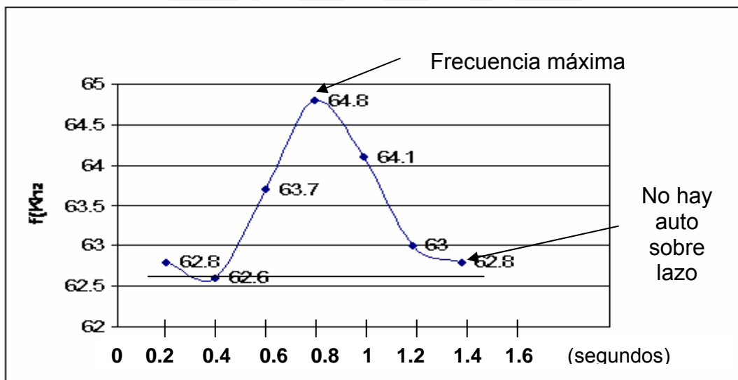
Figura 4.2: Respuesta en frecuencia de presencia auto sobre un 60% del lazo.
