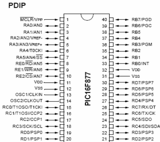
Figura 3.2: Vista del Microcontrolador PIC 16f877a, en empaque tipo PDIP de 40 pines.
