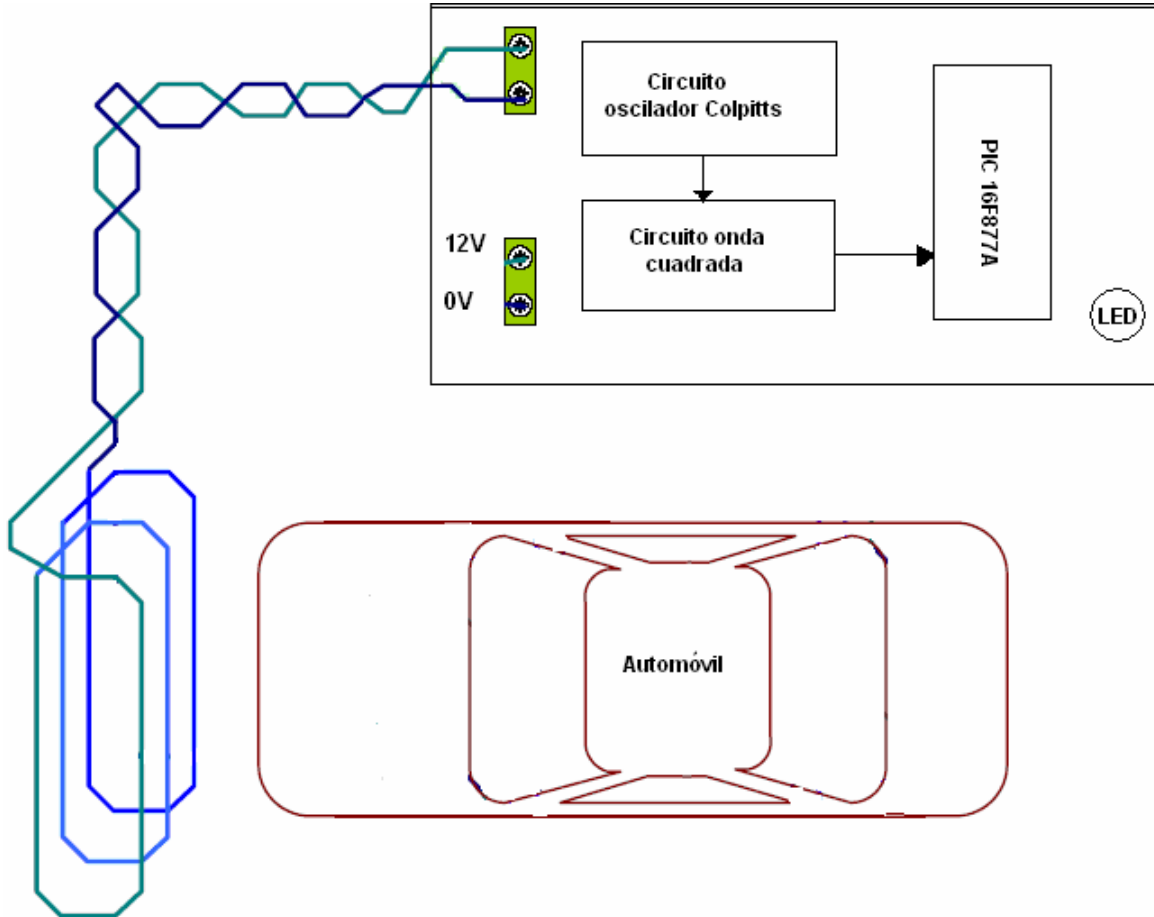
Figura 3.5: Diagrama de bloques de las partes que en conjunto hacen la tarjeta de detección.
