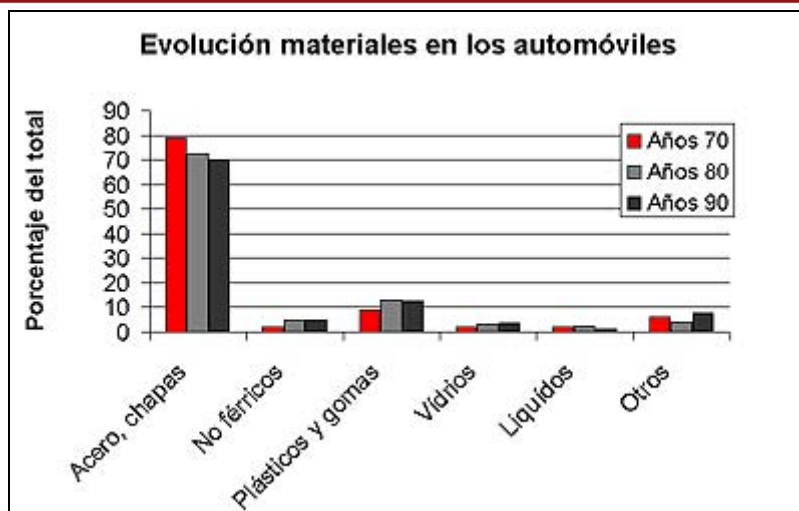
Figura 1.2: Evolución de los materiales en los vehículos.
