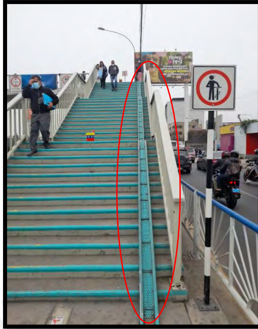
Figura 24. Rampa de acceso para bicicletas en el puente peatonal
