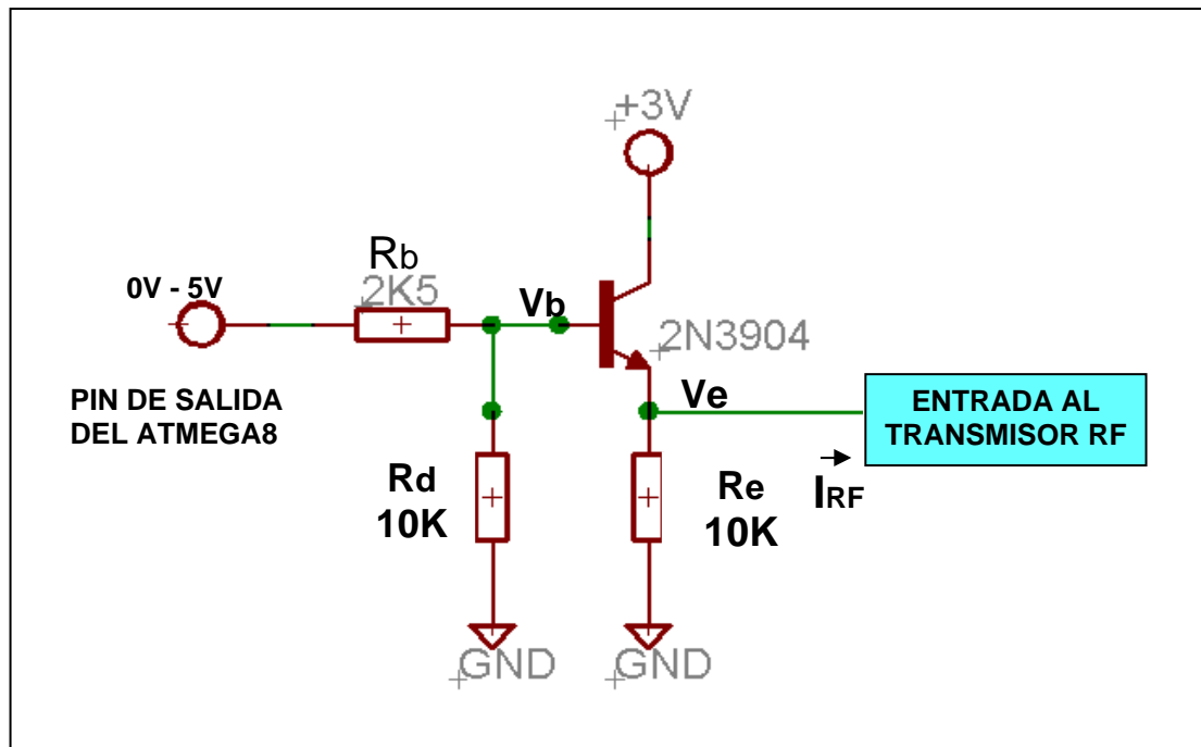
Figura 3.7 Acoplamiento de voltaje en el transmisor
