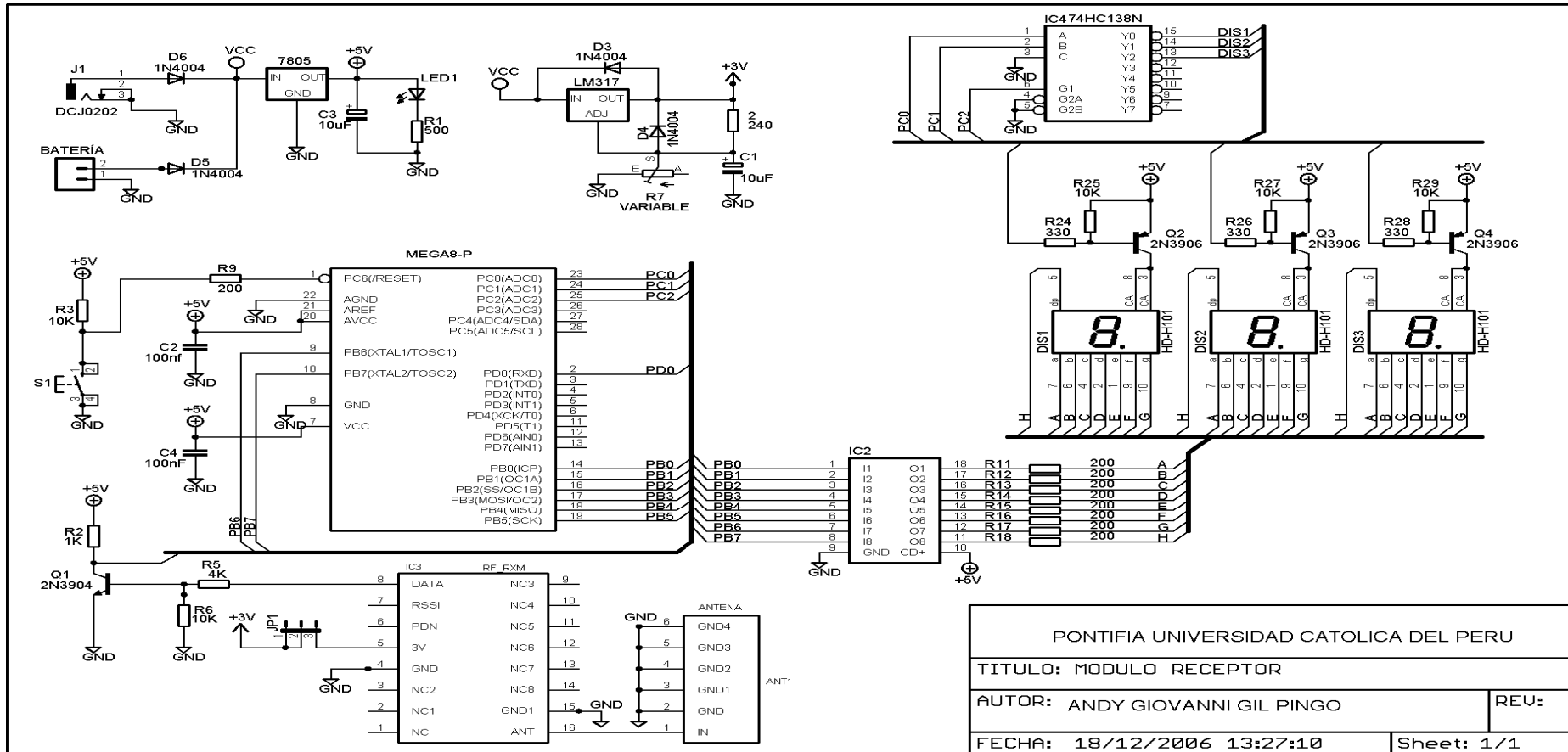
Figura 4.2 Diagrama esquemático completo del módulo receptor
