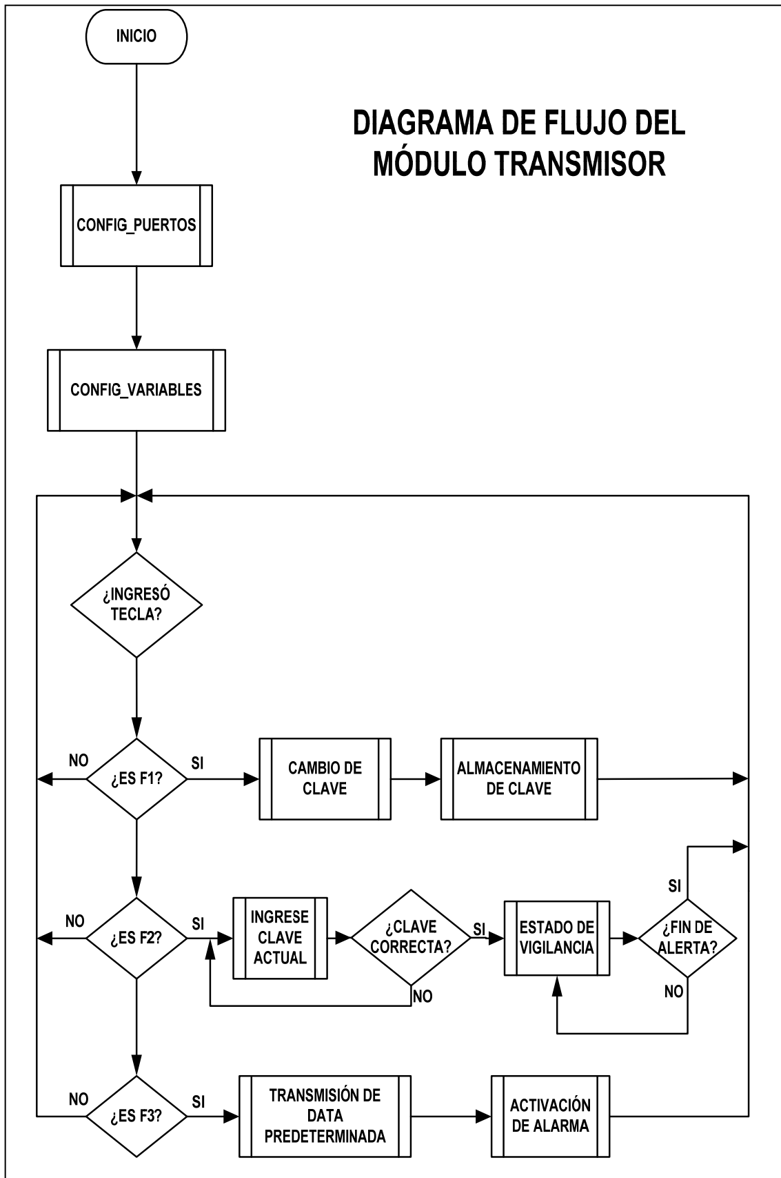
Figura 3.1 Diagrama de flujo del módulo transmisor
