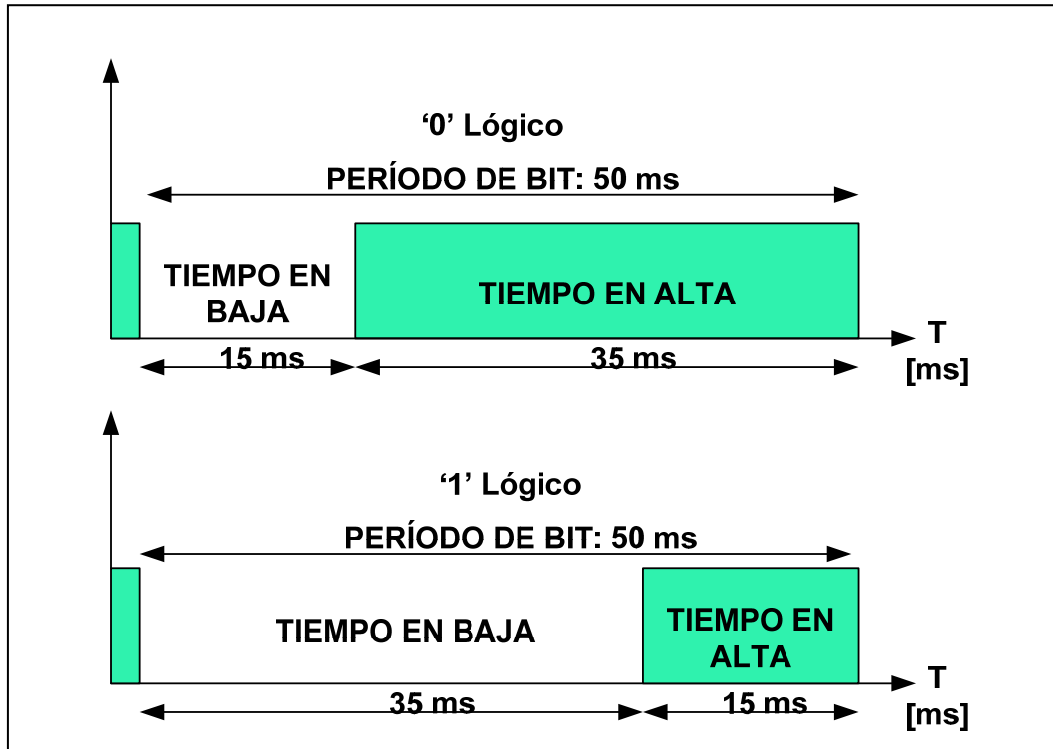
Figura 3.5 Representación del bit en la transmisión
