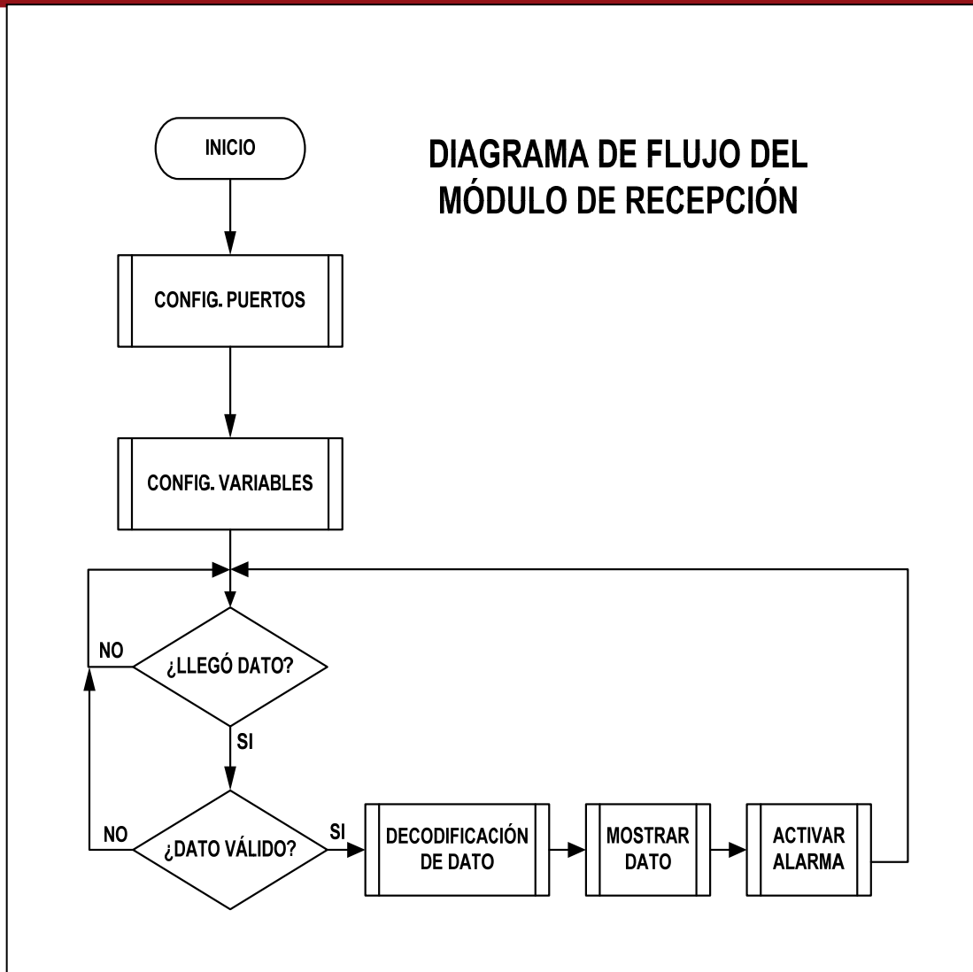
Figura 3.3 Diagrama de flujo del módulo receptor
