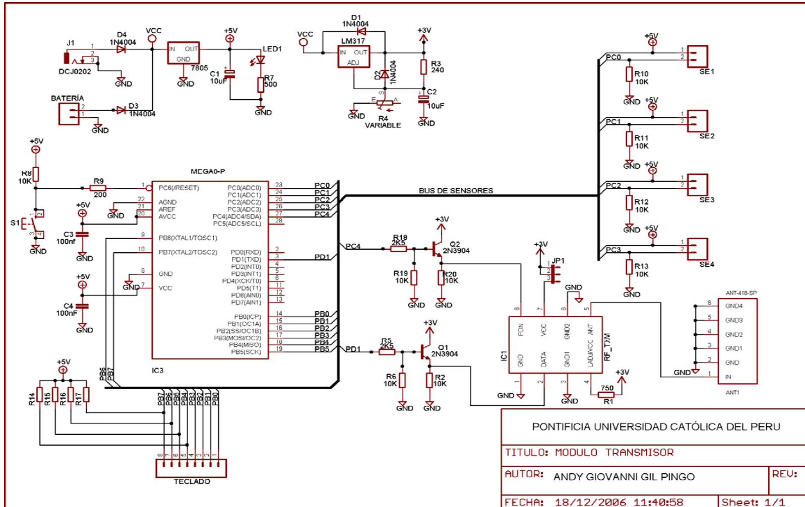
Figura 4.1 Diagrama esquemático completo del módulo transmisor
