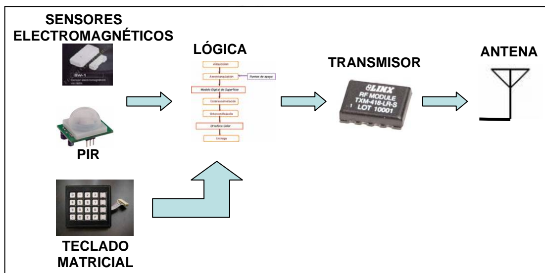
Figura 3.1 Diagrama de bloques del módulo de transmisión
