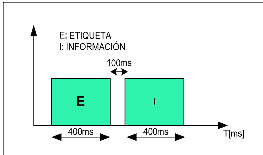
Figura 3.9 Representación de la trama
