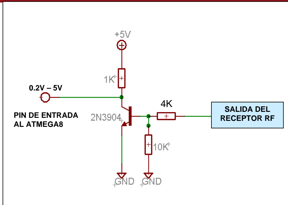
Figura 3.8 Acoplamiento de voltaje en el receptor
