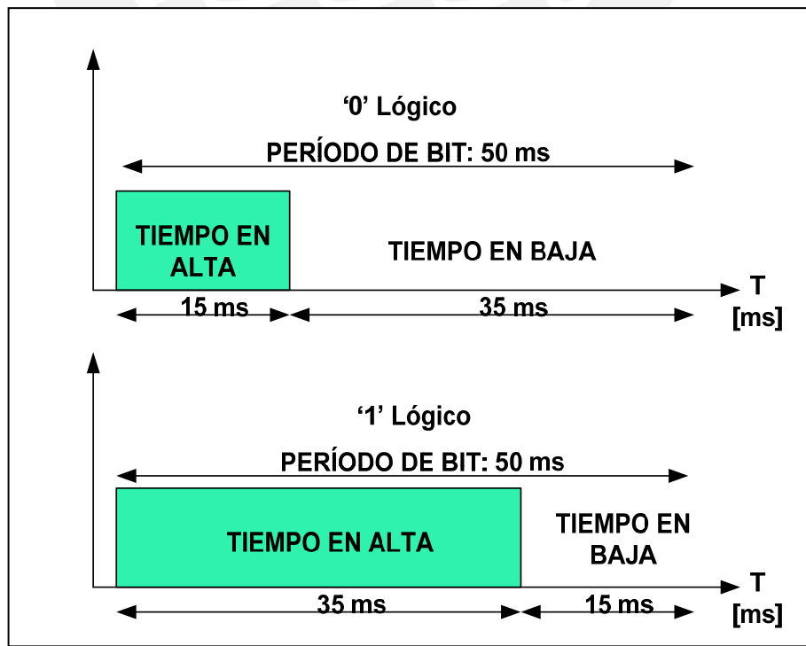
Figura 3.6 Representación del bit en la recepción
