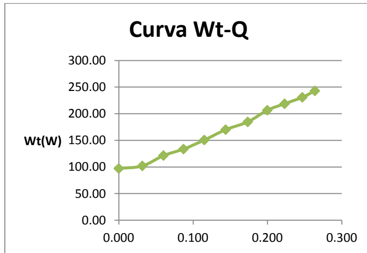
Curva característica a 2600 rpm.
