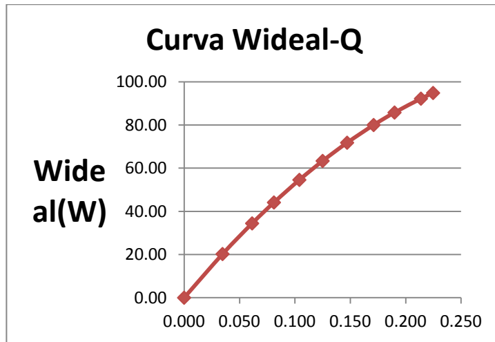
Curva característica a 2200 rpm.
