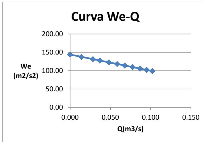
Curva característica a 1000 rpm.
