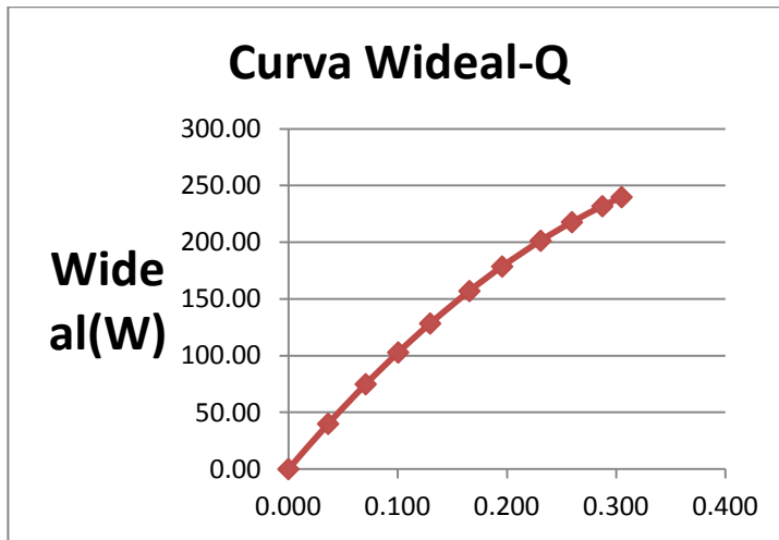
Curva característica a 3000 rpm.
