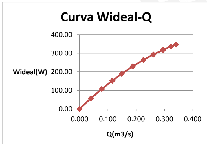
Curva característica a 3400 rpm.
