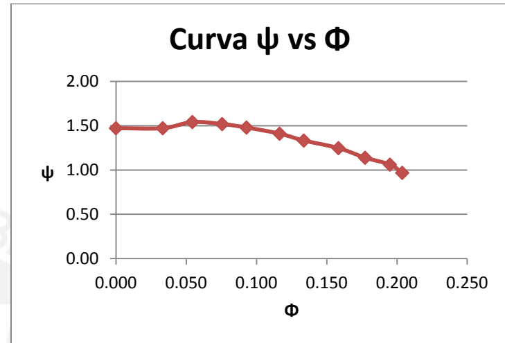
Curva característica a 2000 rpm.
