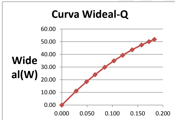
Curva característica a 1800 rpm.
