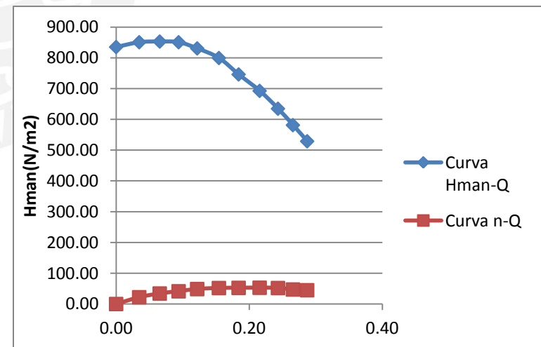
Curva característica a 2800 rpm.
