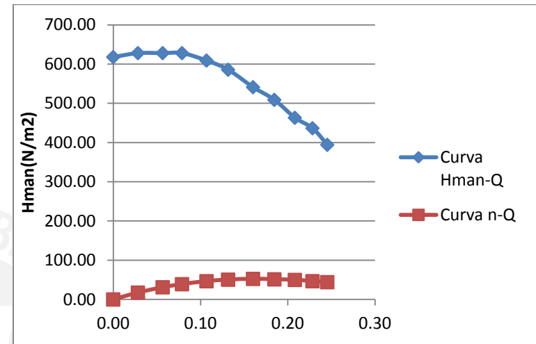
Curva característica a 2400 rpm.
