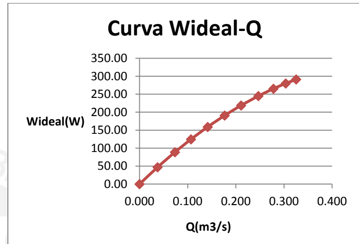
Curva característica a 3200 rpm.
