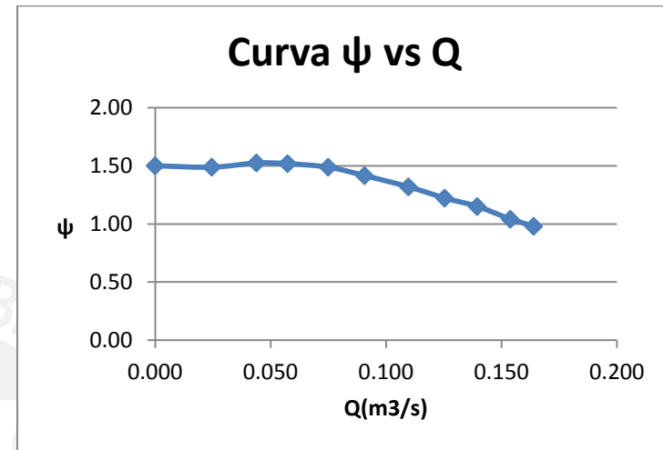
Curva característica a 1600 rpm.
