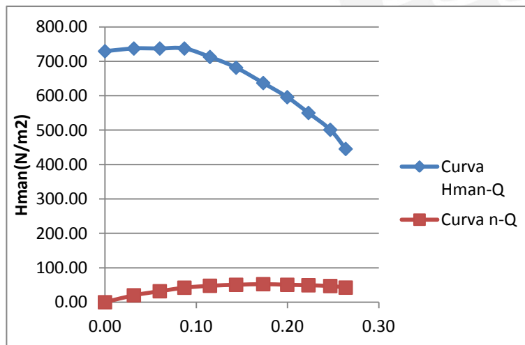
Curva característica a 2600 rpm.
