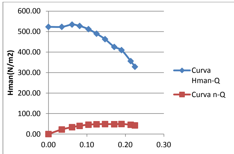
Curva característica a 2200 rpm.
