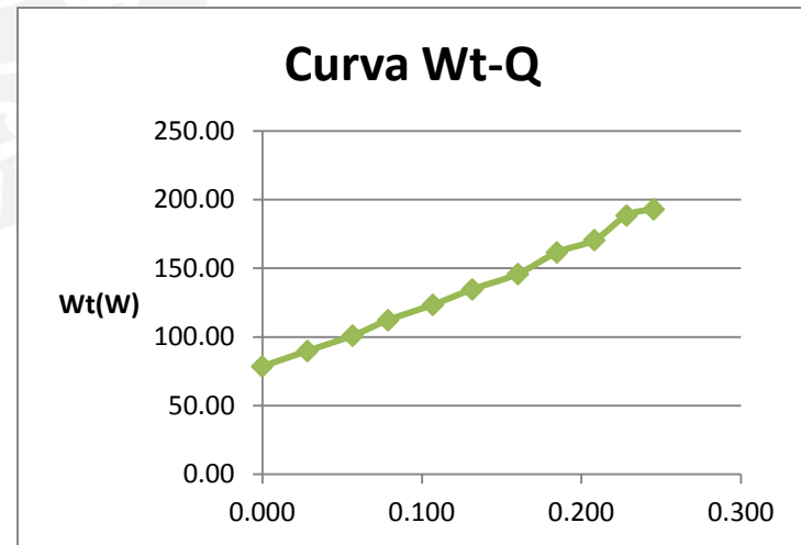
Curva característica a 2400 rpm.
