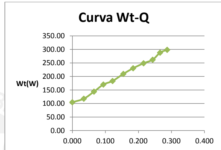
Curva característica a 2800 rpm.
