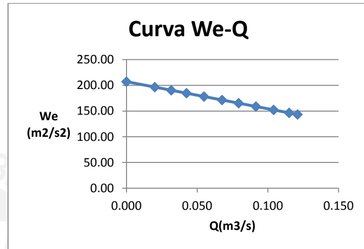
Curva característica a 1200 rpm.
