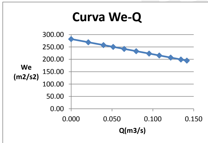
Curva característica a 1400 rpm.
