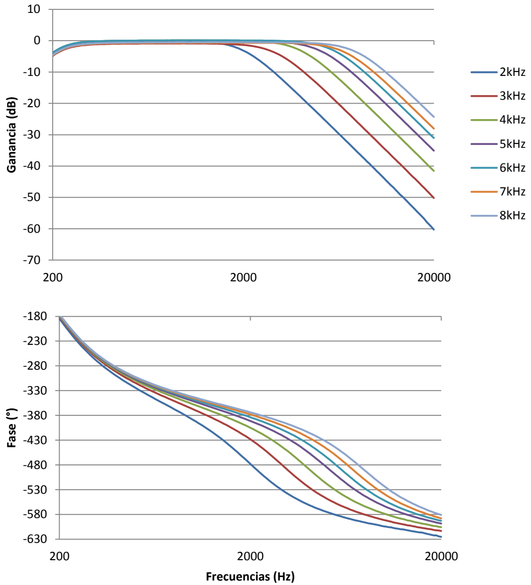
Figura A5.15: Alineamiento Butterworth Tercer Orden
