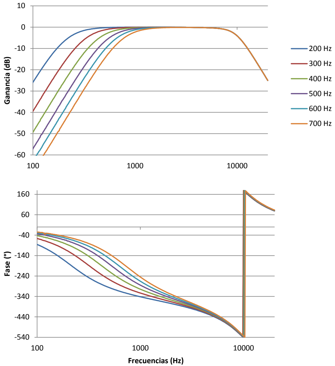
Figura A5.12: Alineamiento Linkwitz-Riley Cuarto Orden
