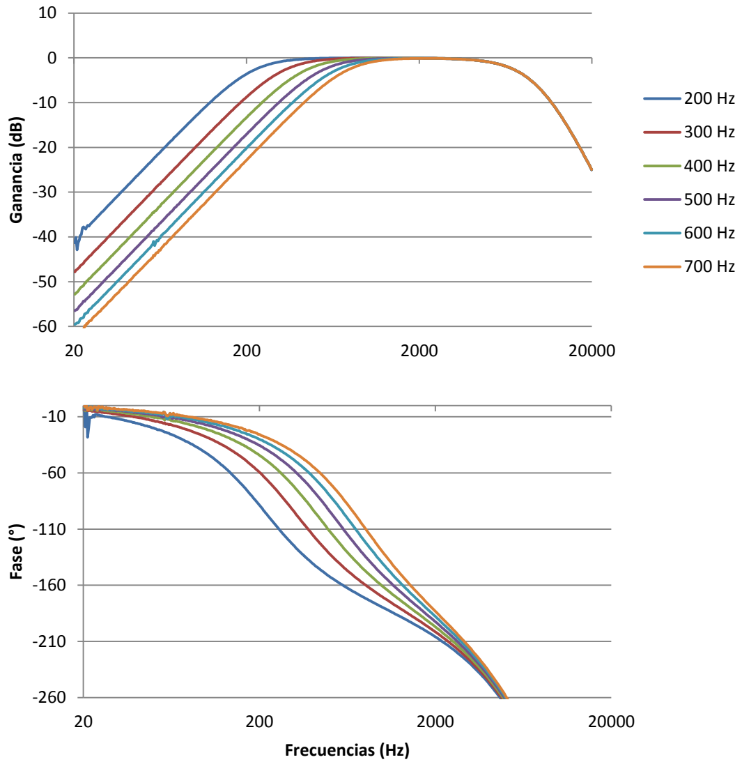
Figura A5.8: Alineamiento Butterworth Segundo Orden
