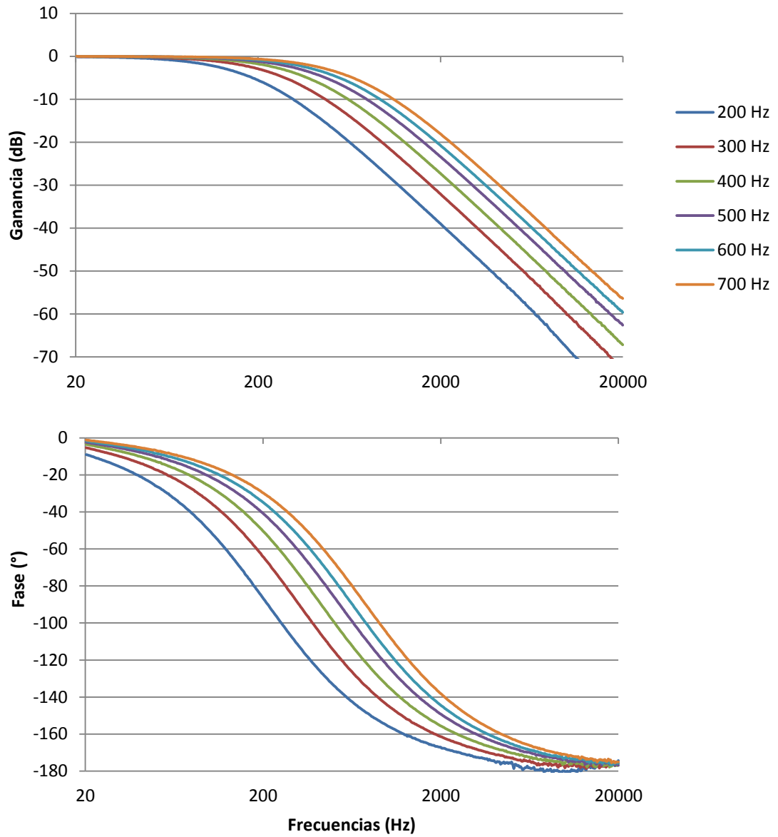
Figura A5.5: Alineamiento Linkwitz-Riley Segundo Orden
