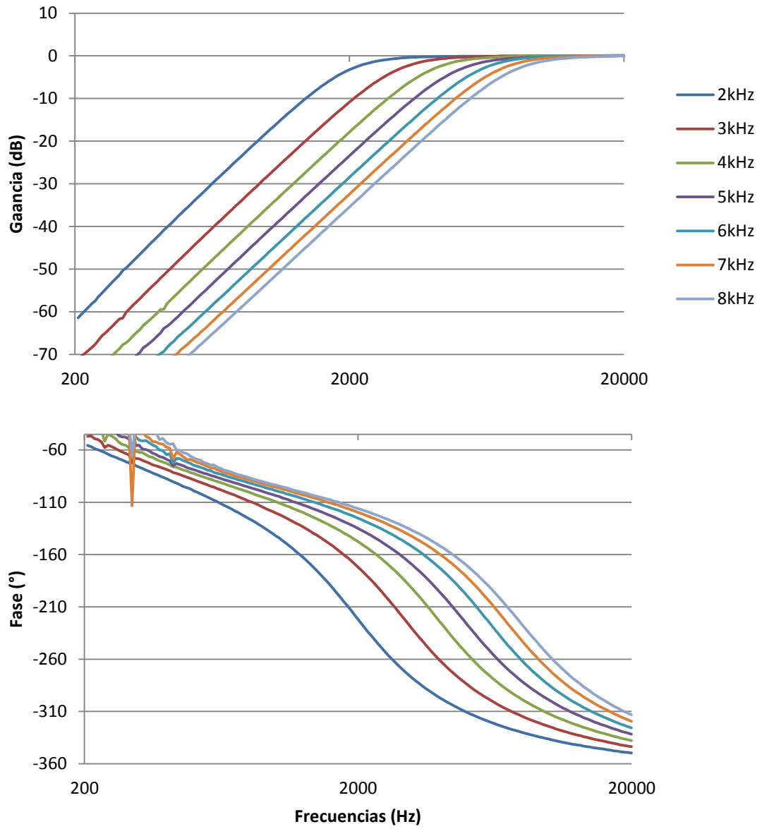
Figura A5.21: Alineamiento Butterworth Tercer Orden
