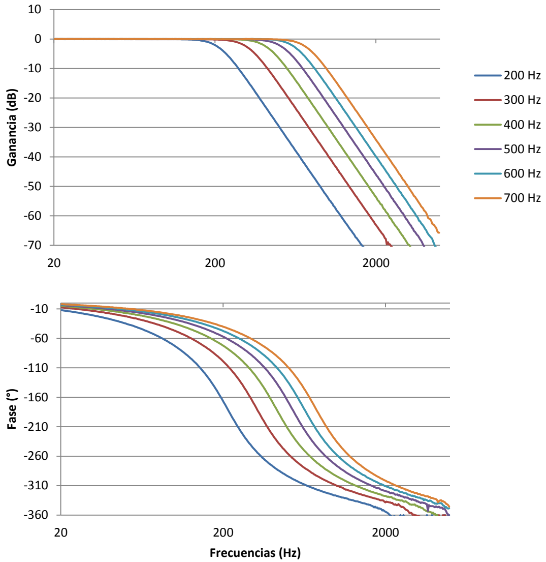
Figura A5.4: Alineamiento Butterworth Cuarto Orden
