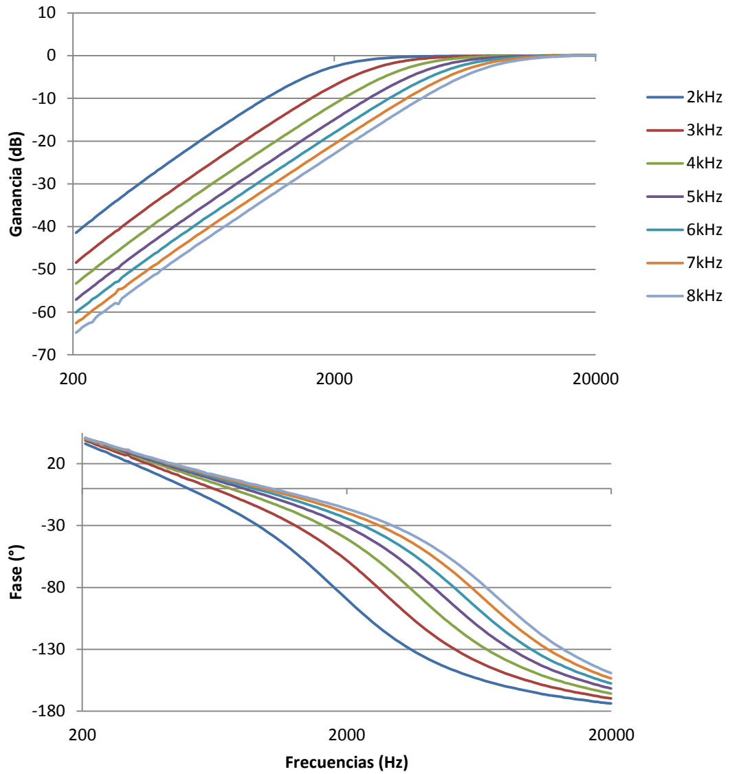
Figura A5.20: Alineamiento Butterworth Segundo Orden
