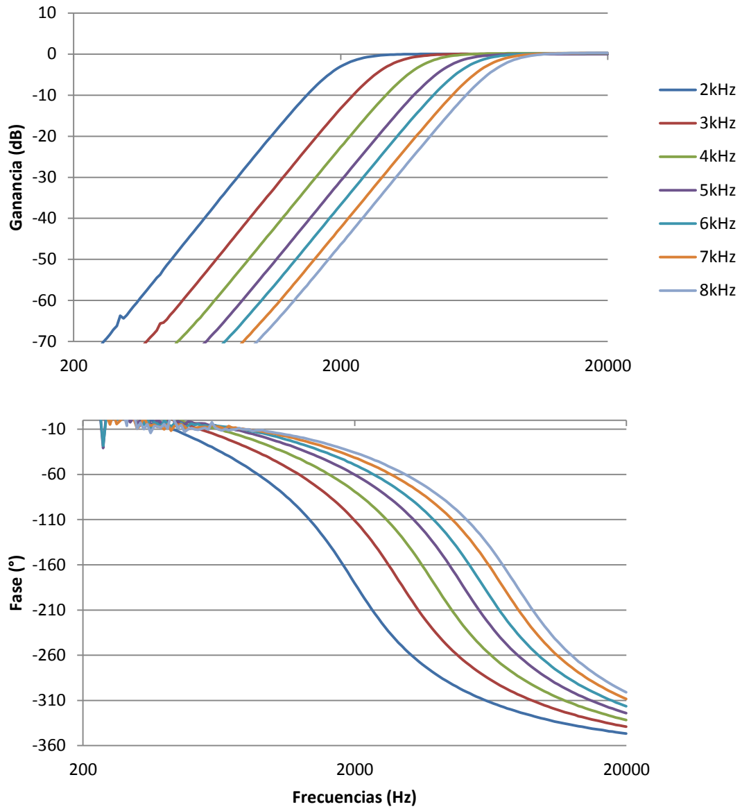
Figura A5.22: Alineamiento Butterworth Cuarto Orden
