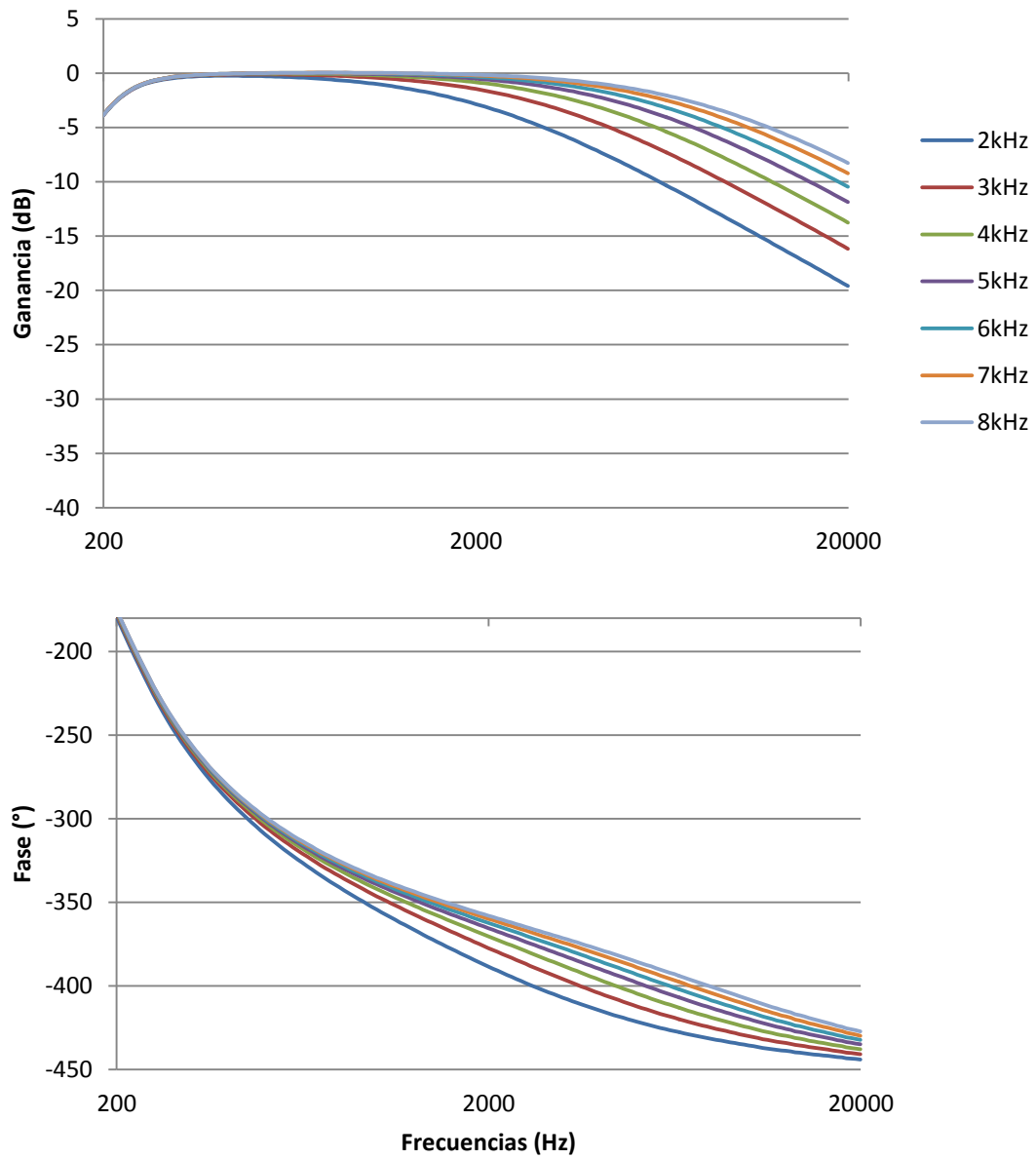
Figura A5.13: Alineamiento Butterworth Primer Orden
