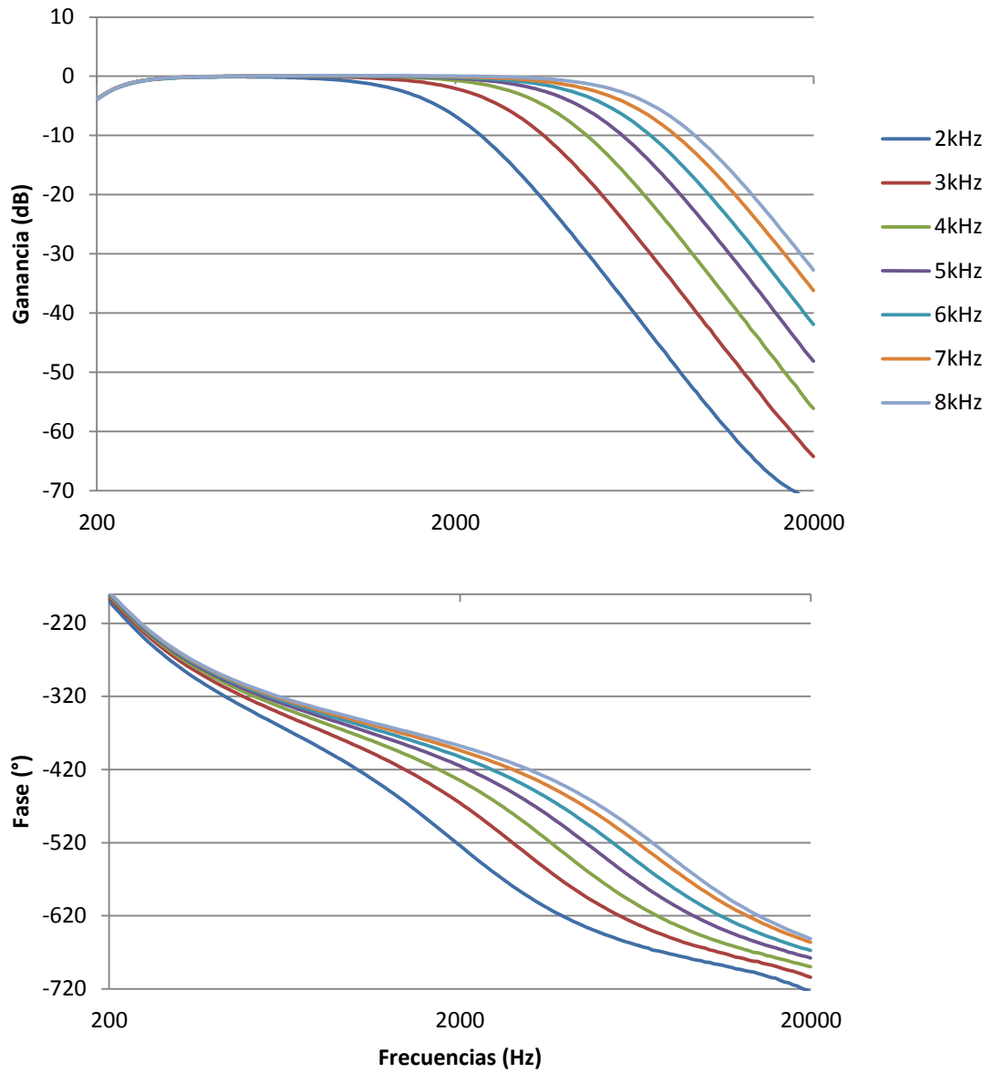
Figura A5.18: Alineamiento Linkwitz-Riley Cuarto Orden
