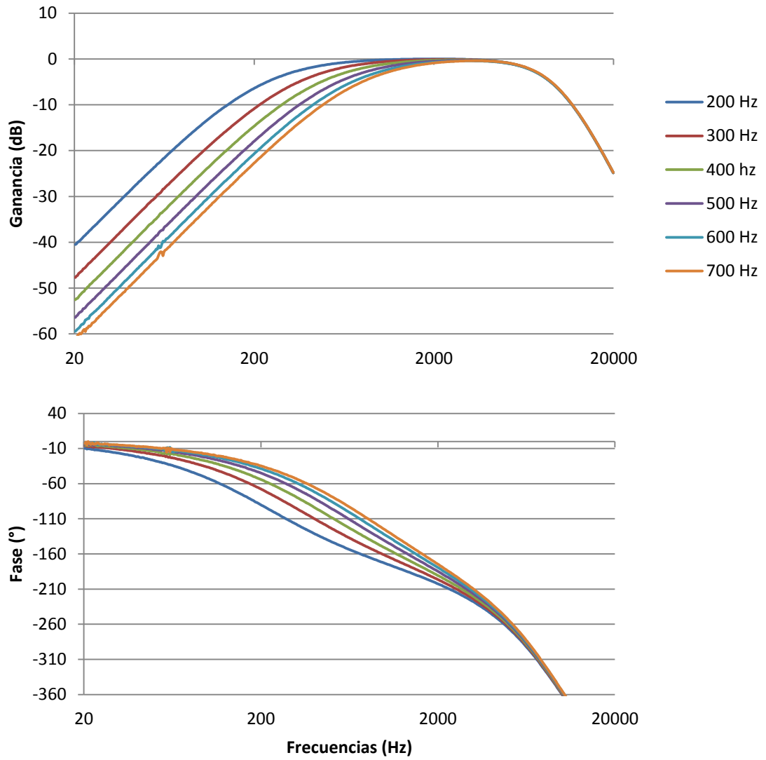
Figura A5.11: Alineamiento Linkwitz-Riley Segundo Orden
