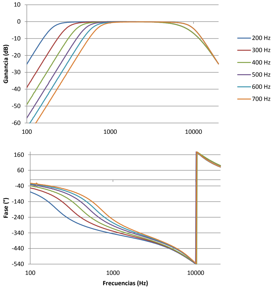
Figura A5.10: Alineamiento Butterworth Cuarto Orden
