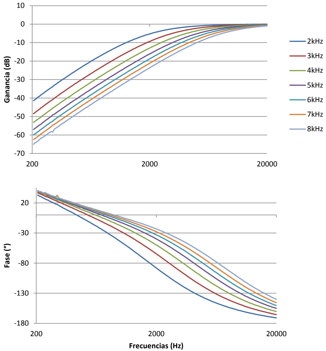
Figura A5.23: Alineamiento Linkwitz-Riley Segundo Orden
