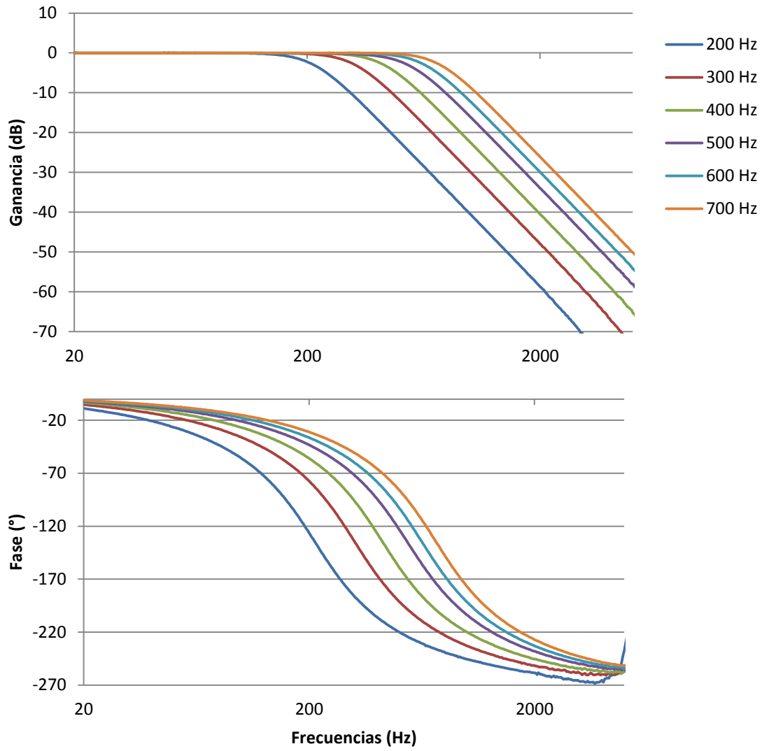
Figura A5.3: Alineamiento Butterworth Tercer Orden
