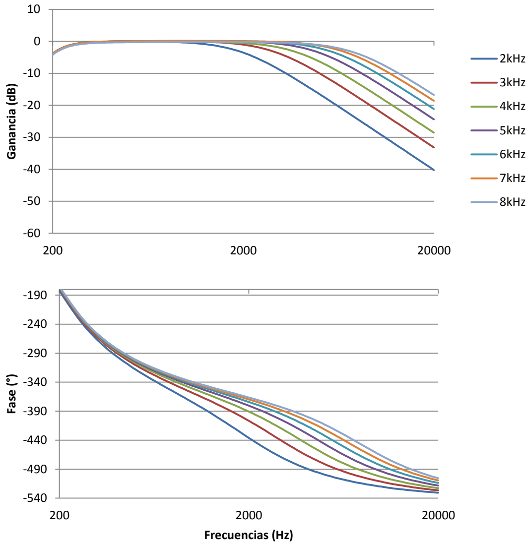
Figura A5.14: Alineamiento Butterworth Segundo Orden
