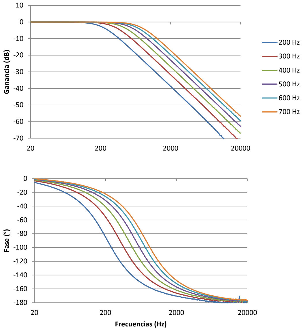
Figura A5.2: Alineamiento Butterworth Segundo Orden
