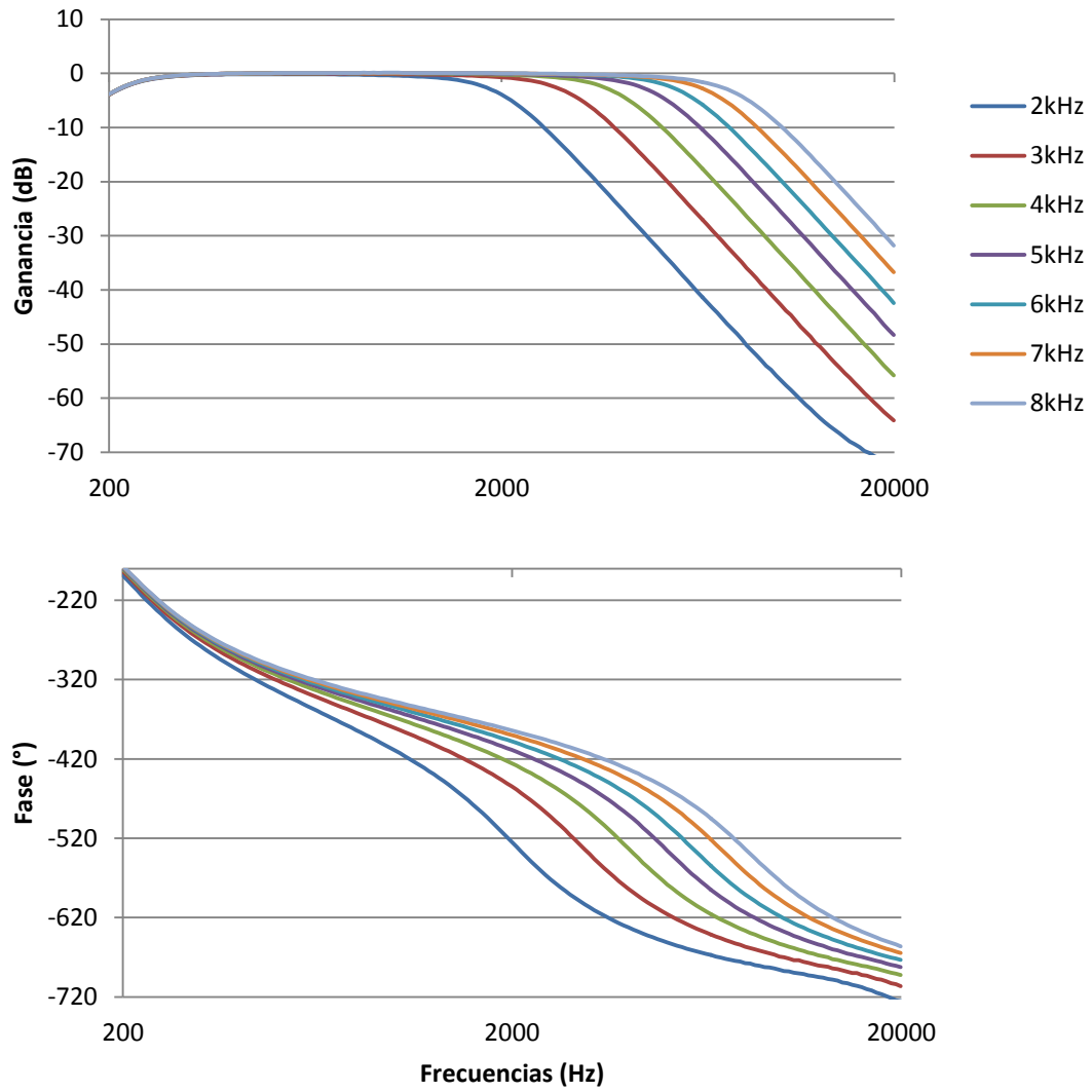
Figura A5.16: Alineamiento Butterworth Cuarto Orden
