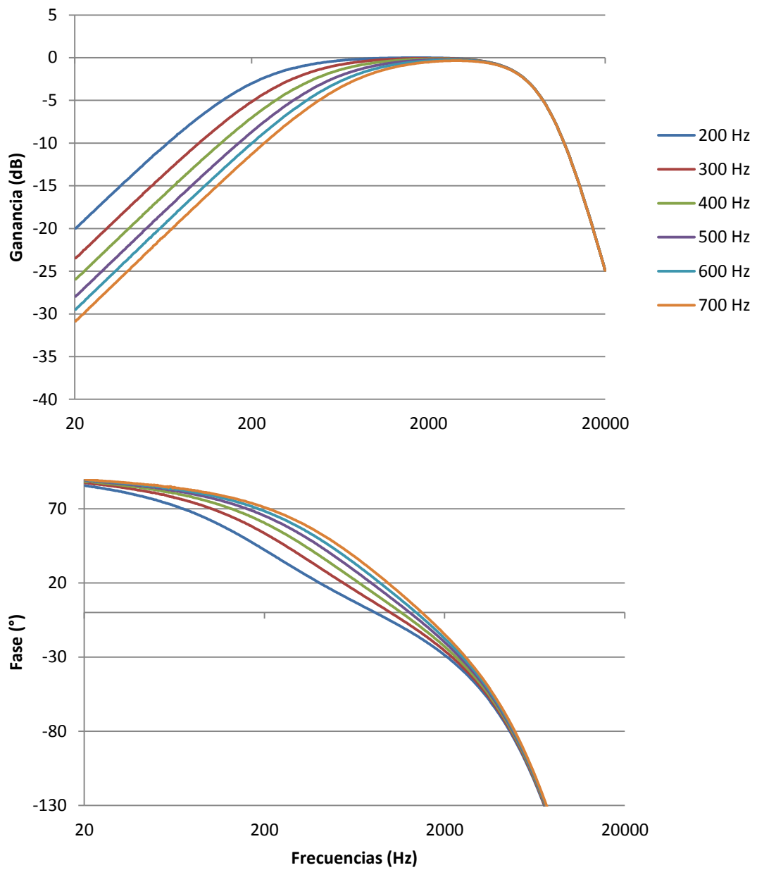
Figura A5.7: Alineamiento Butterworth Primer Orden
