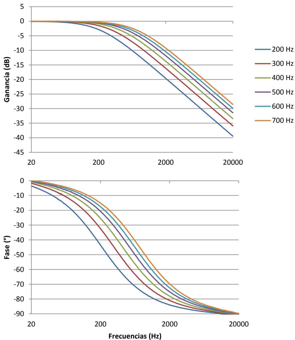
Figura A5.1: Alineamiento Butterworth Primer Orden
