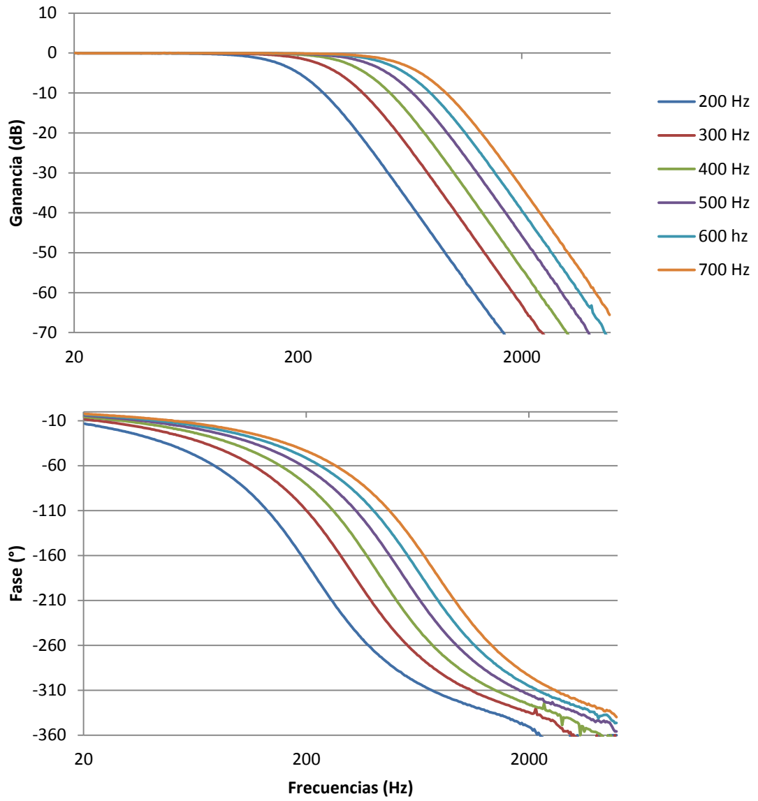
Figura A5.6: Alineamiento Linkwitz-Riley Cuarto Orden
