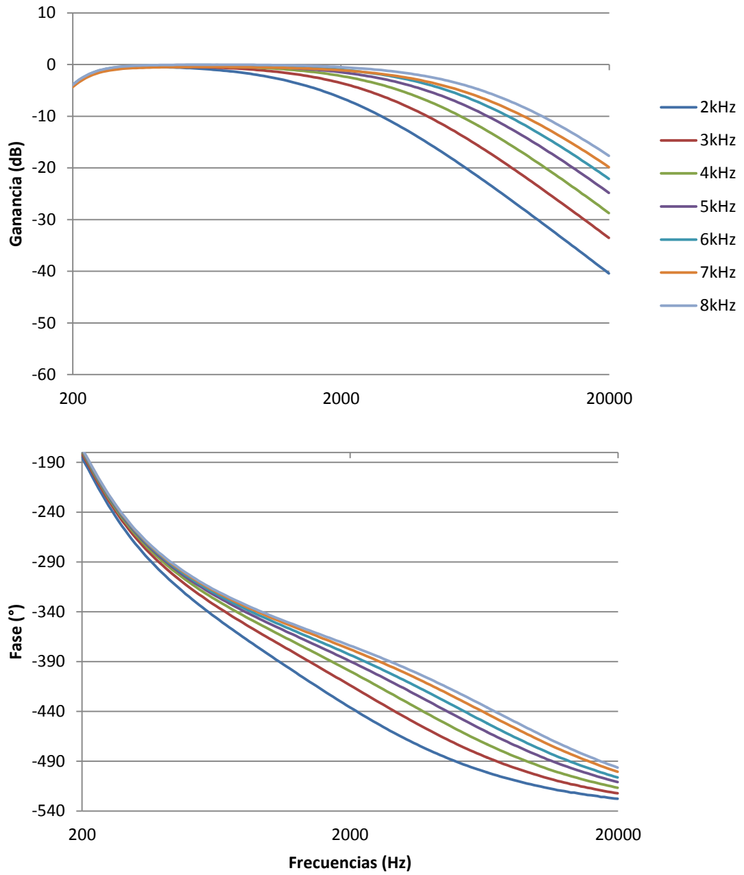
Figura A5.17: Alineamiento Linkwitz-Riley Segundo Orden
