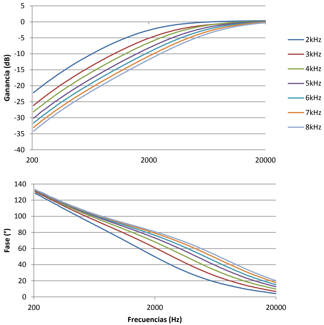
Figura A5.19: Alineamiento Butterworth Primer Orden
