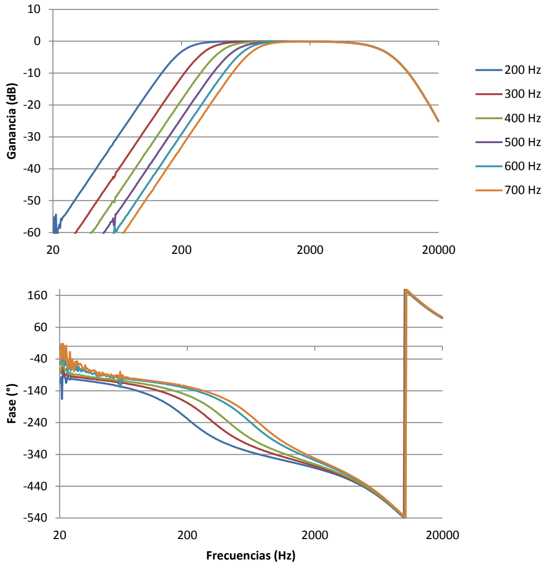
Figura A5.9: Alineamiento Butterworth Tercer Orden
