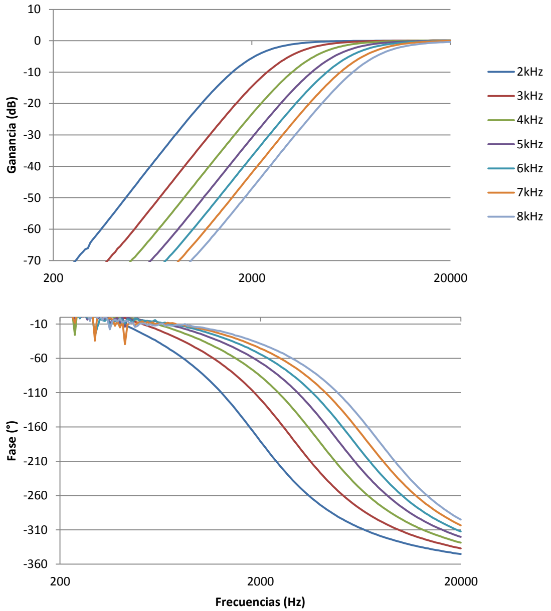
Figura A5.24: Alineamiento Linkwitz-Riley Cuarto Orden
