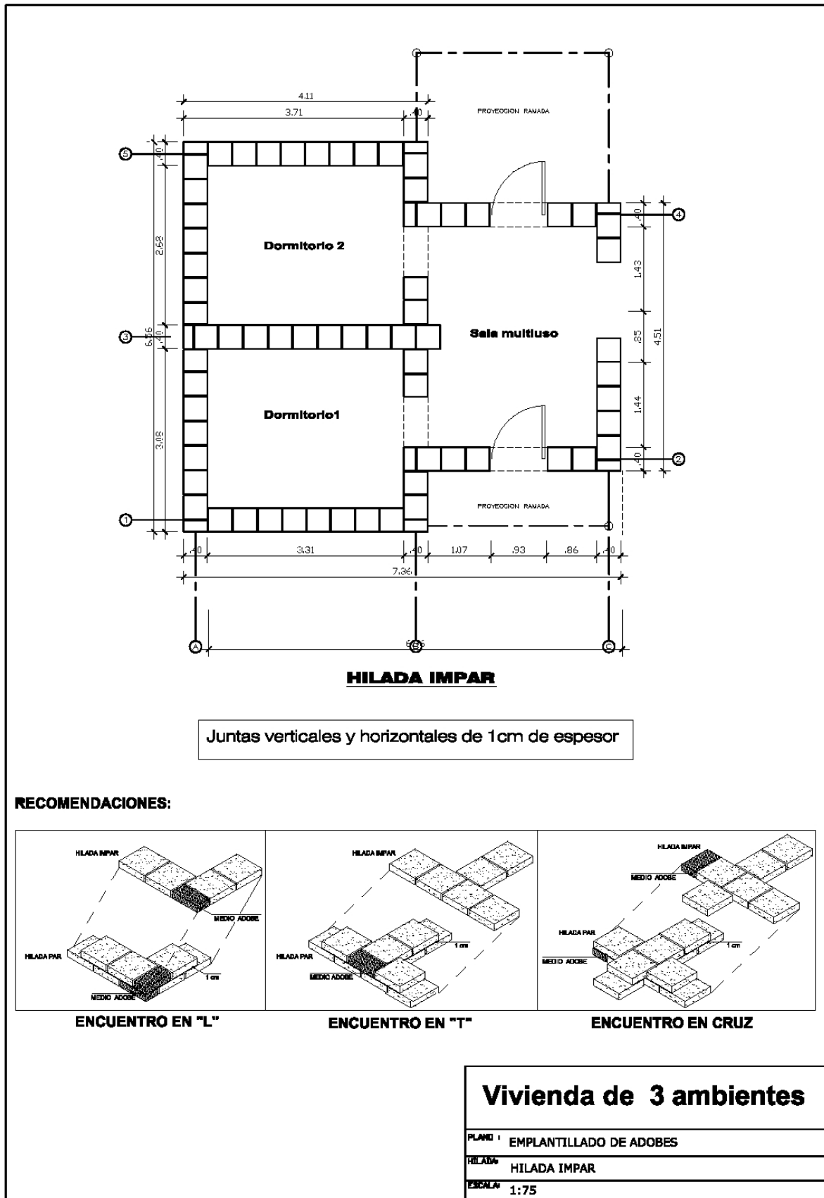
Figura 3.9. Ejemplo de planos de construcción para una vivienda de tres ambientes.
