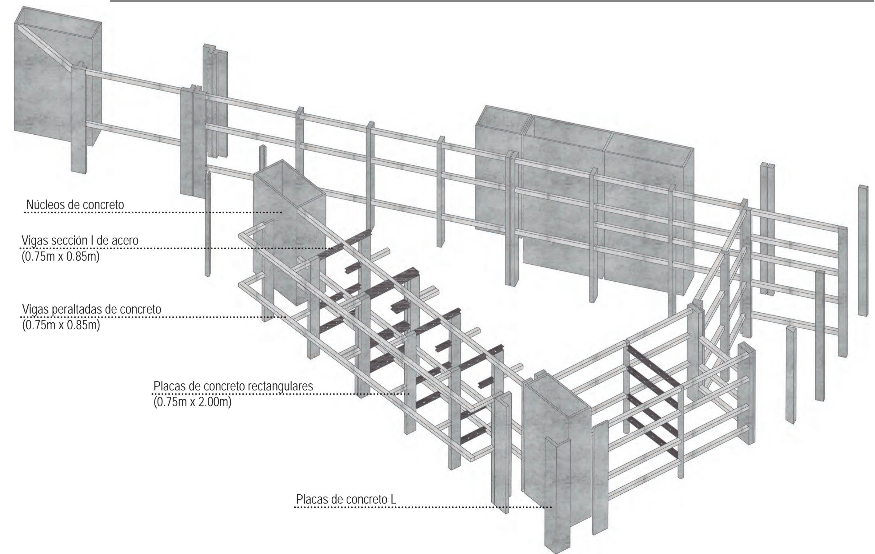
Sección D- Detalle 1:75 Barra Transparente: Materializa arquitectónicamente el concepto de reinserción social penitenciaria y pone en evidencia la importante relación sensorial que necesita el proyecto y su ubicación en un entorno urbano vivo.
