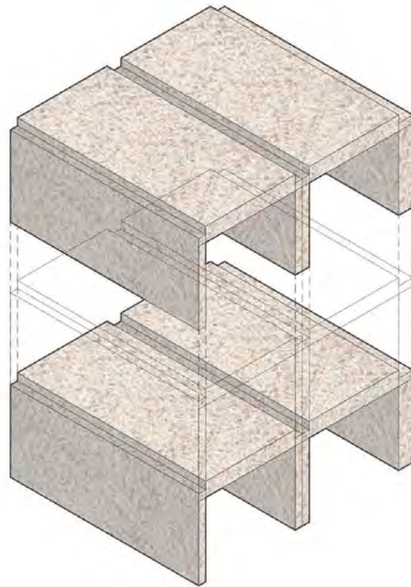
Anclaje y Modulación de Nichos Base Nicho Base prefabricado en concreto terrazado. 2m x 1.1m x 92.5cm, e:5cm
