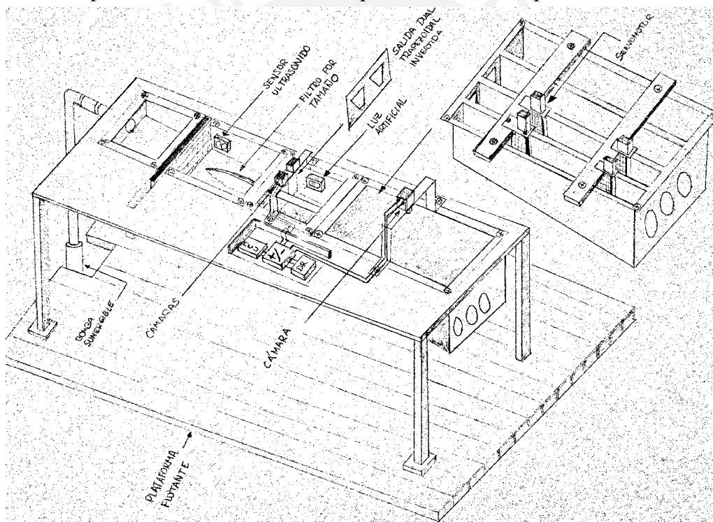
Fig. 2.4 – Dibujo de concepto de solución N° 1.
