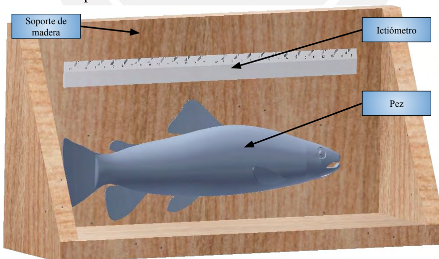
Fig. 1.5 – Herramienta de medición manual para peces.
