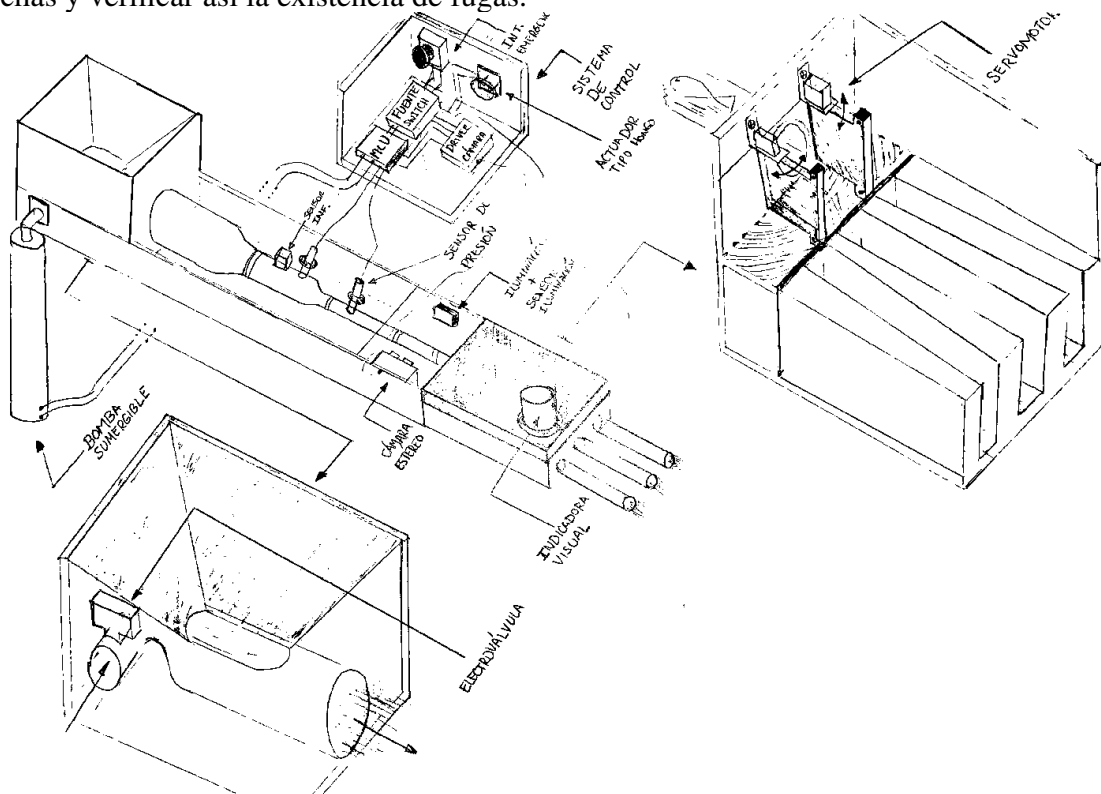
Fig. 2.5 – Dibujo de concepto de solución N° 2.
