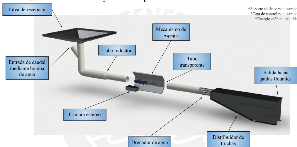
Fig. 2.6 – Concepto virtual del concepto de solución N° 2.
