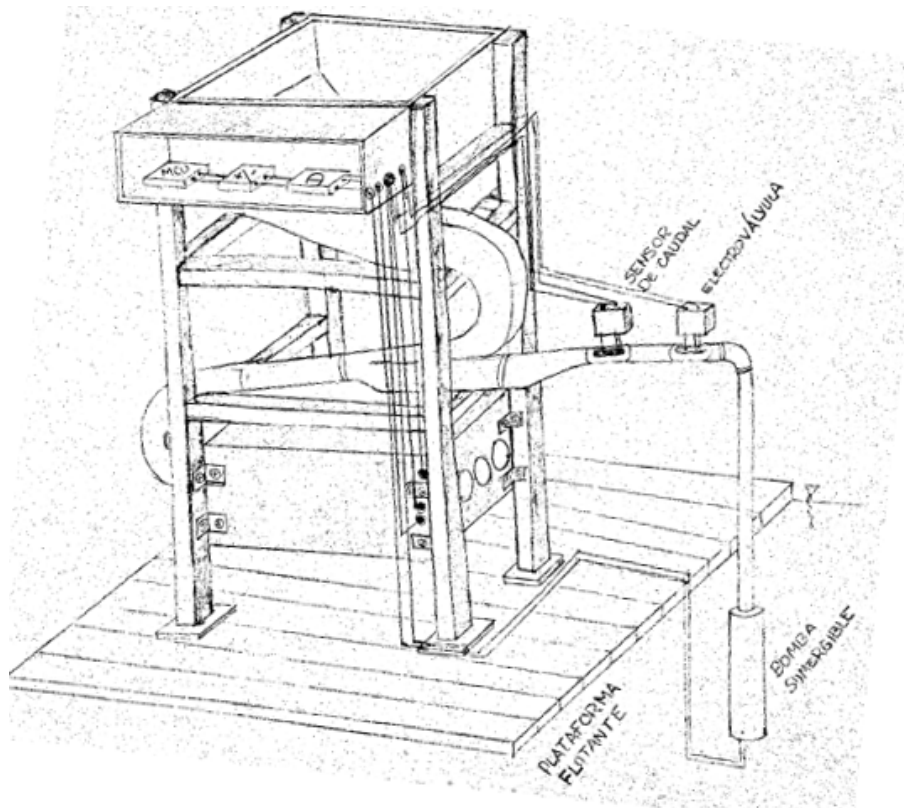
Fig. 2.7 – Dibujo de concepto de solución N° 3.
