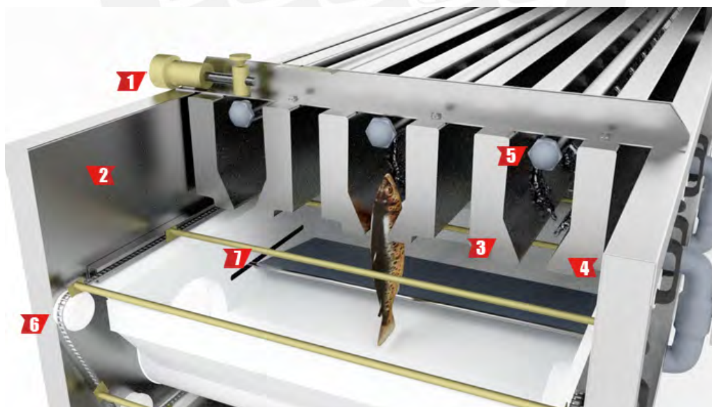
Fig. 1.23 – Clasificadoras automáticas para peces de origen francés.
