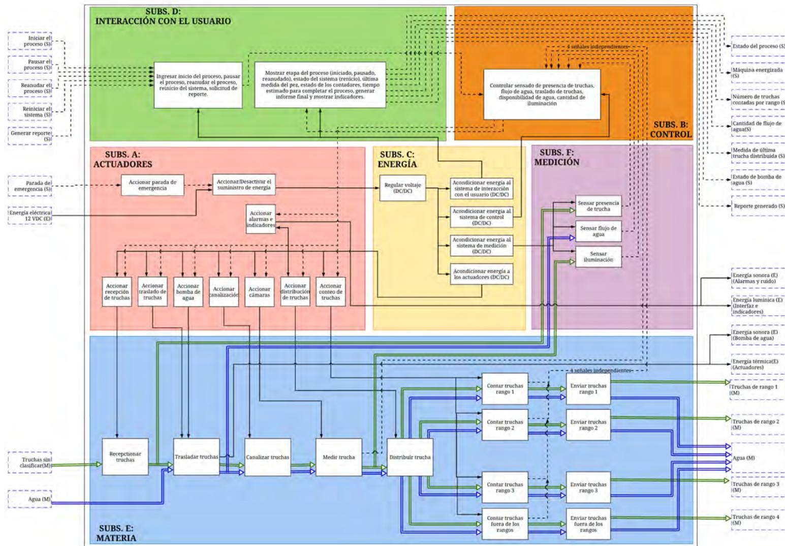
Fig. 2.2 – Estructura global de funciones.
