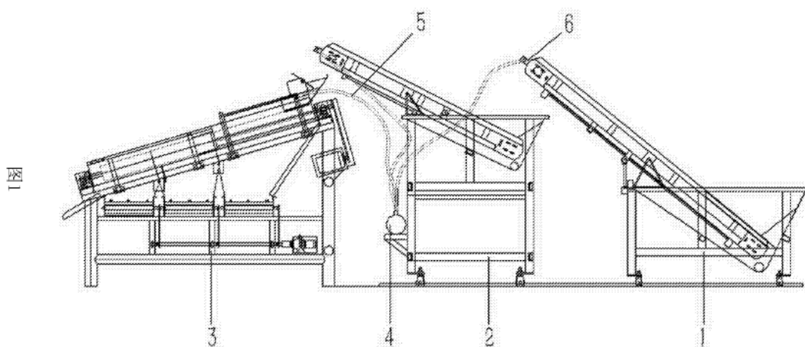
Fig. 1.19 – Clasificadora automática de peces de origen chino.
