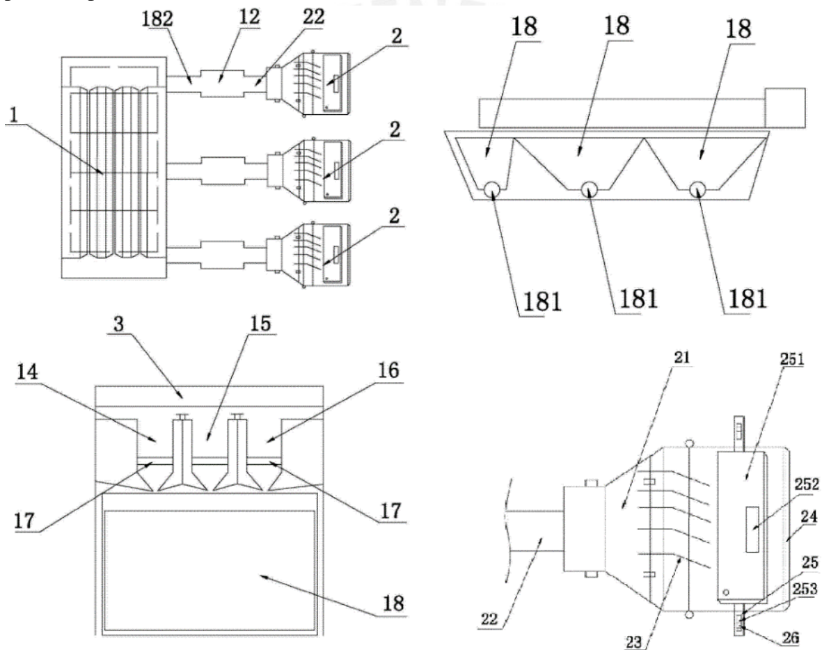
Fig. 1.20 – Clasificadora automática de peces de origen chino.
