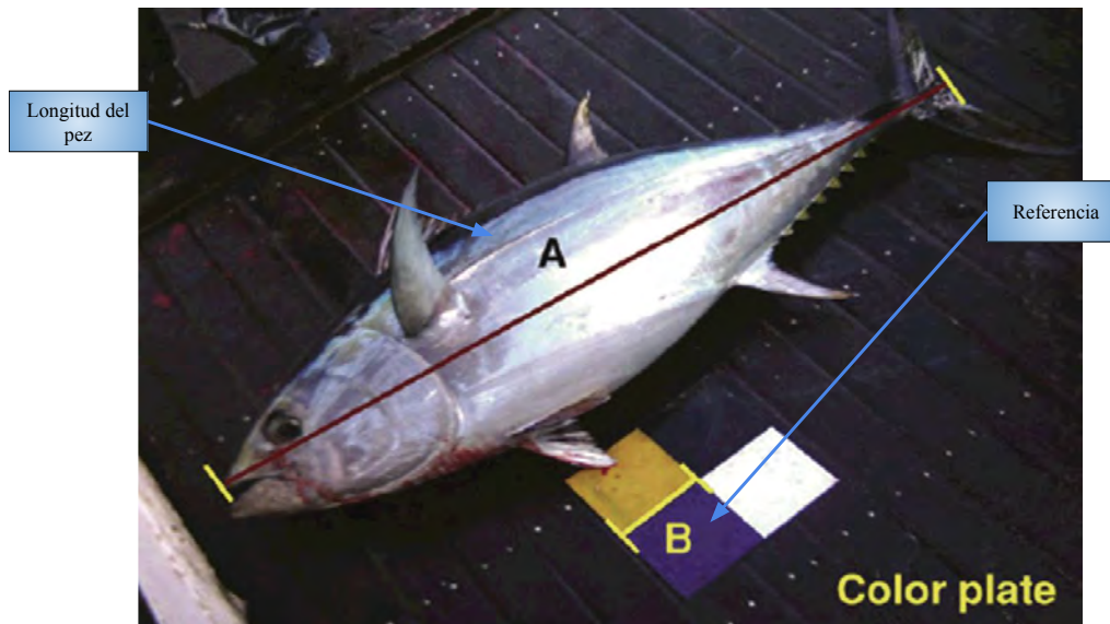
Fig. 1.15 – Usando la relación entre A y B para calcular la longitud del pez.
