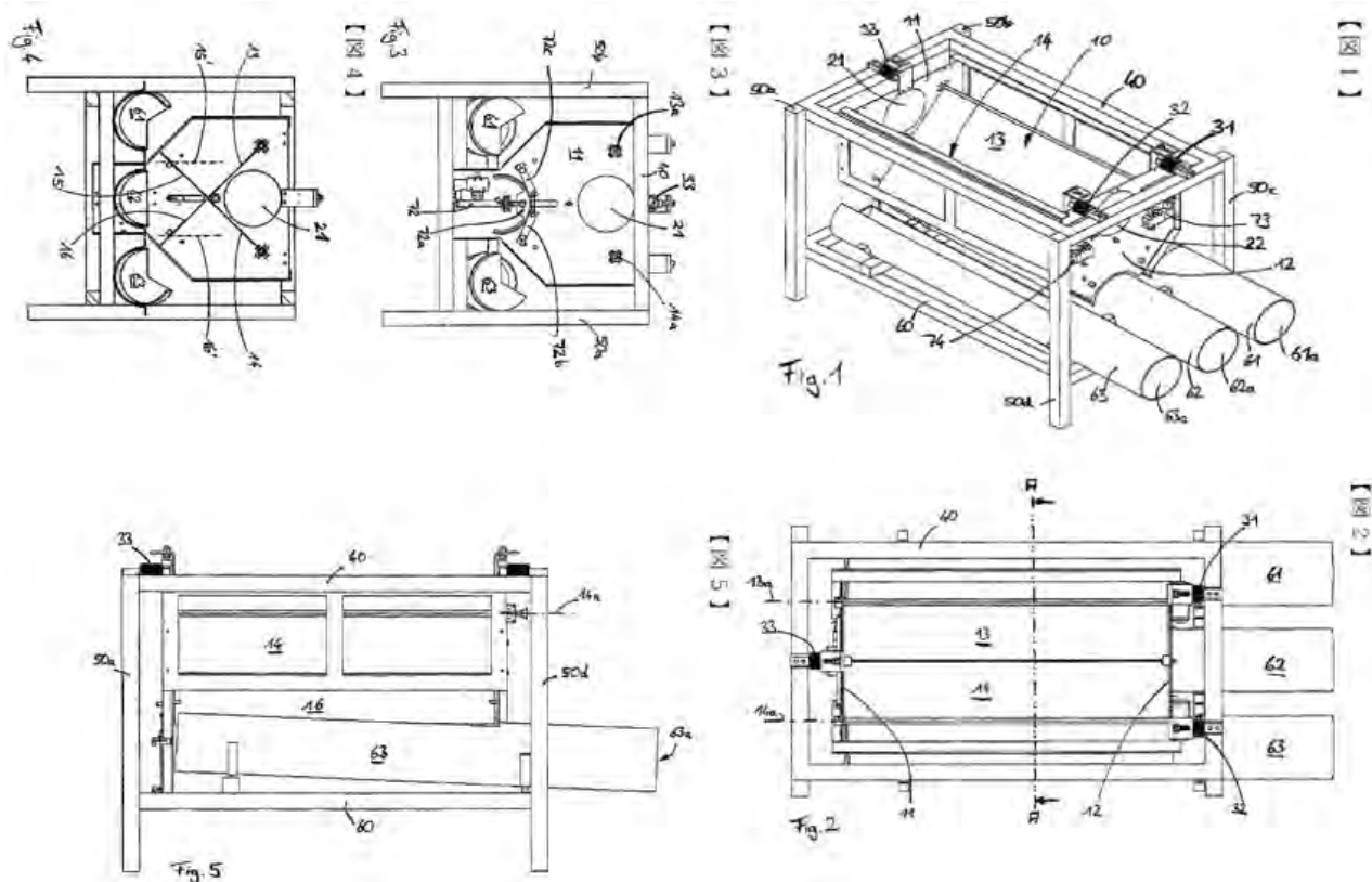
Fig. 1.18 – Clasificadora automática de peces de origen japonés.
