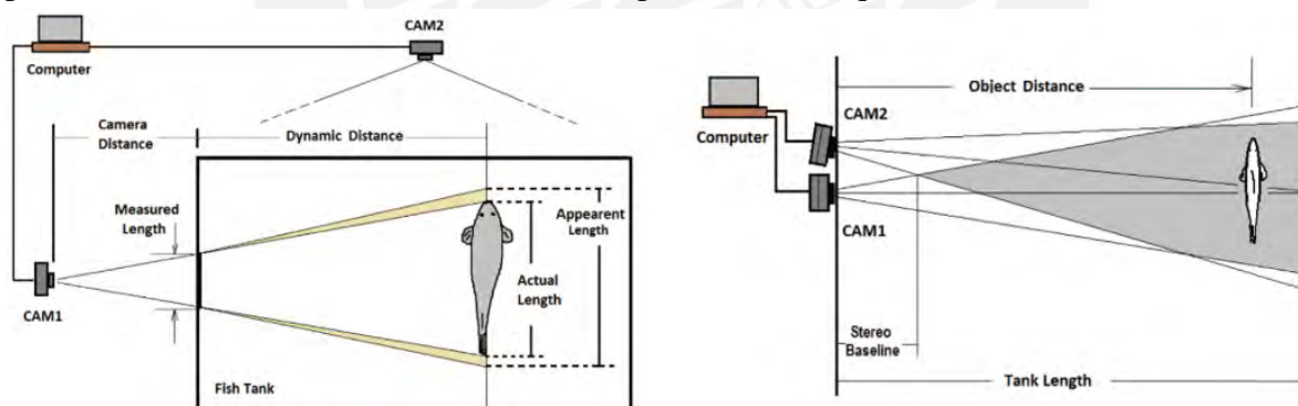
Fig. 1.8 – Medición de peces dentro de estanques con cámaras ortogonales y estéreo.
