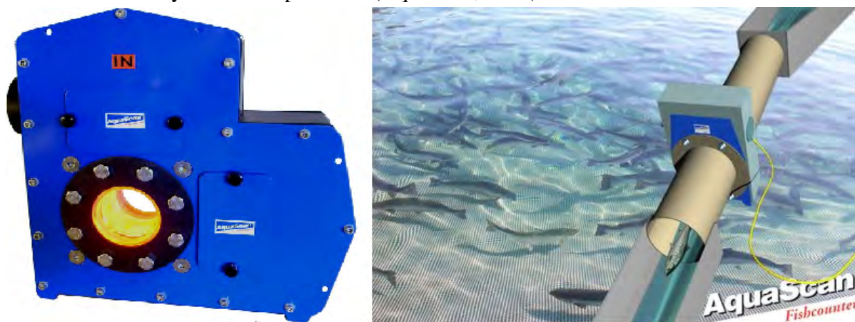
Fig. 1.13 – Contador de peces mediante escáneres.
