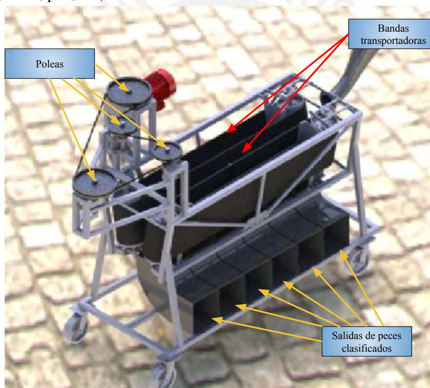
Fig. 1.6 – Máquina seleccionadora de truchas de A. G. V.
