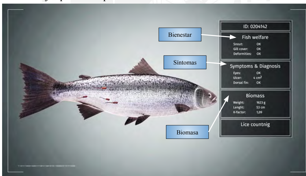
Fig. 1.14 – Extracción de características mediante visión por computadora.
