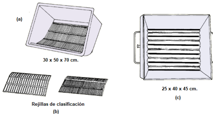
Fig. 1.3 – (a,b,c) Clasificadora de anchura fija, rejillas de clasificación y clasificadora ajustable.
