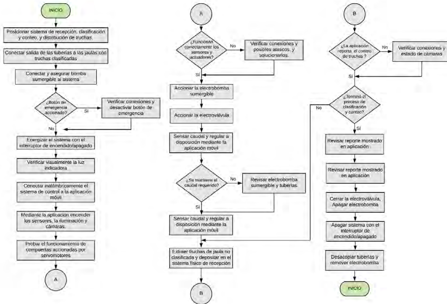
Fig. 2.11 – Flujograma de funcionamiento de la solución óptima.
