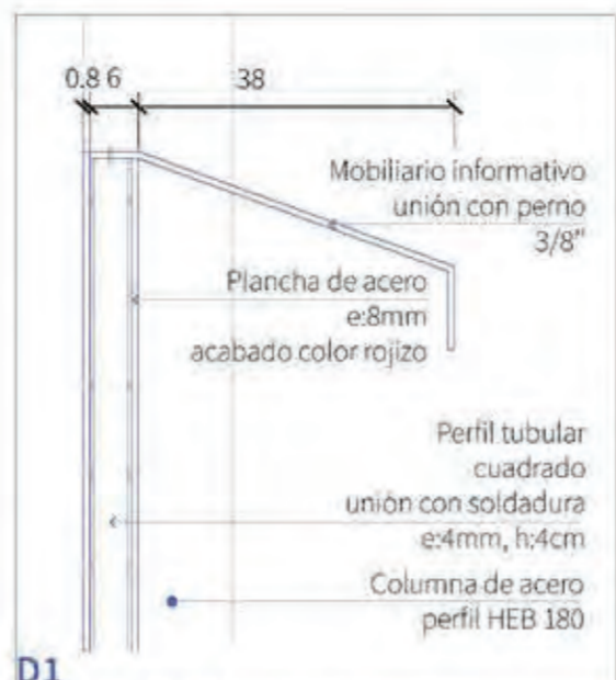
D1 Baranda informativa
