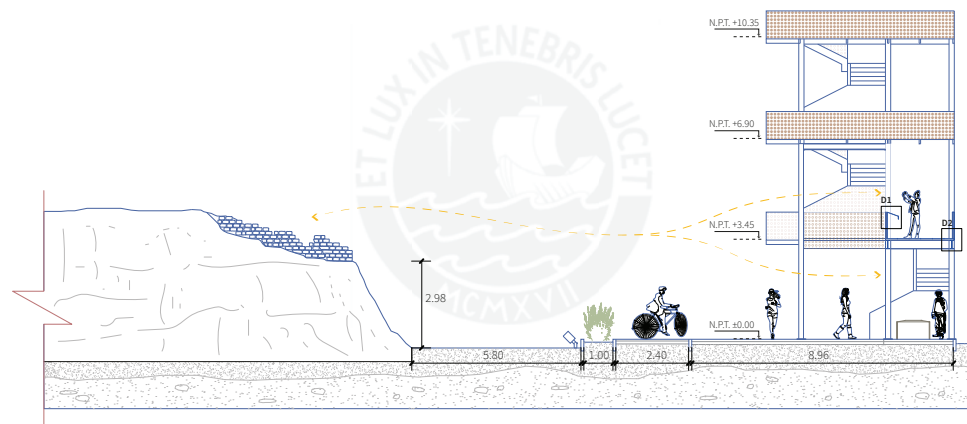
Corte A-A'
