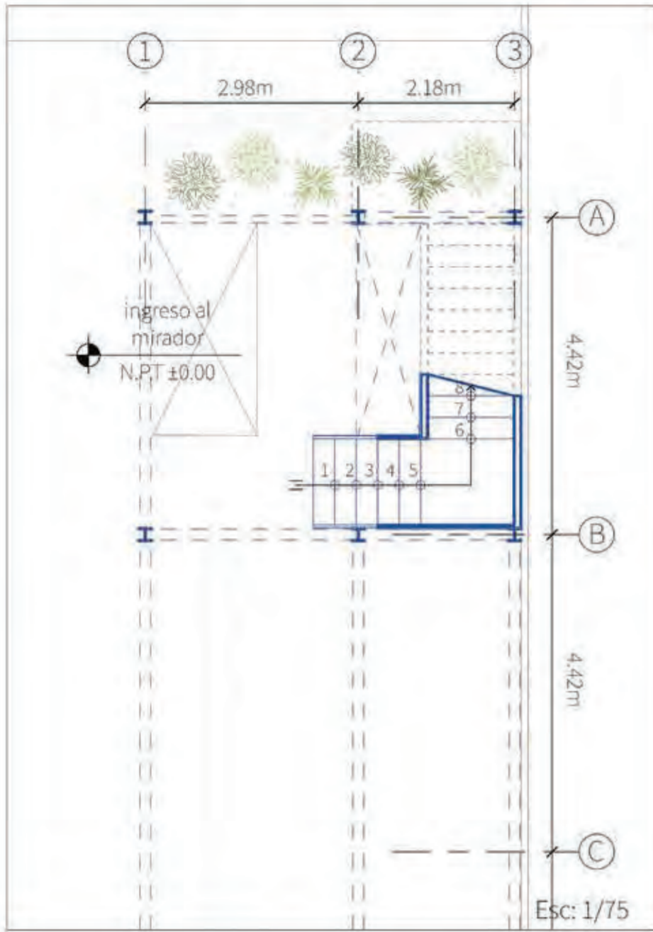
Zoom mirador
