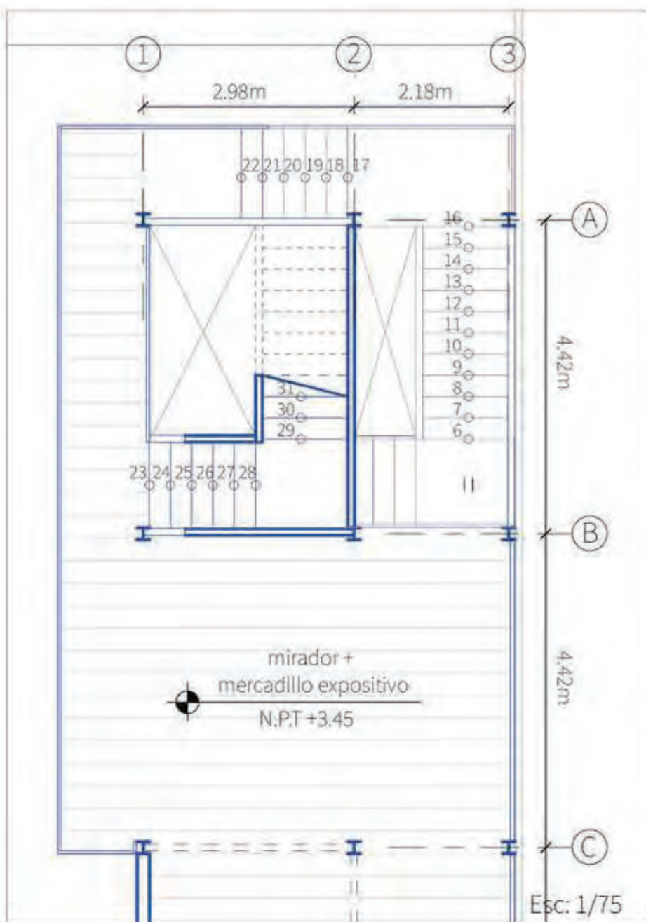
Planta 2
