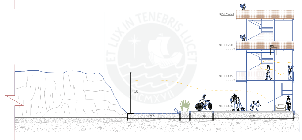
Corte B-B'
