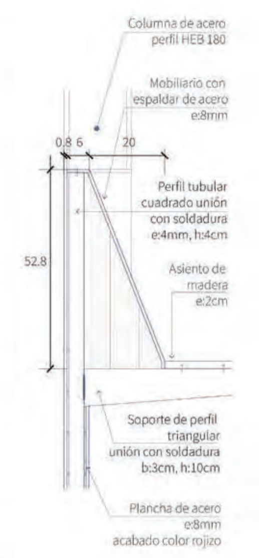
D1 baranda - asiento
