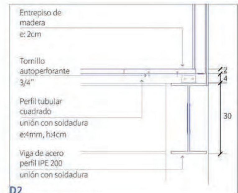
D2 Baranda - entrespiso
