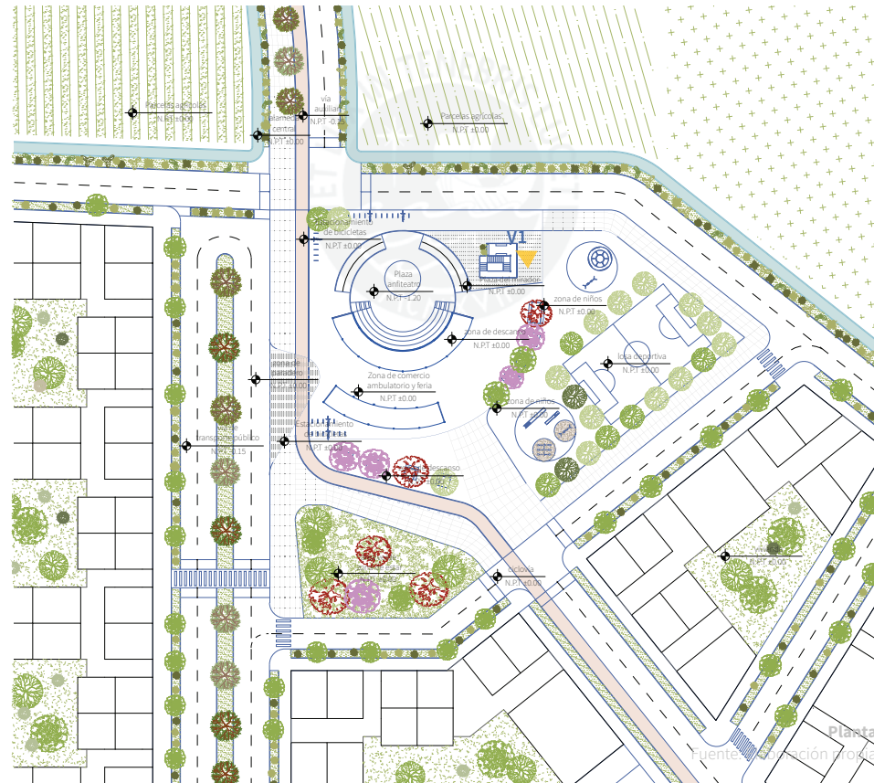
Planta general
