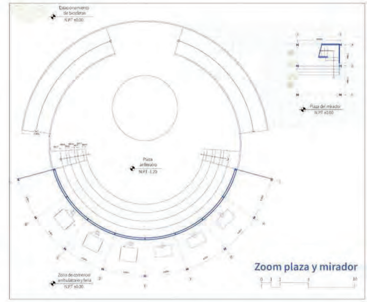
Planta 2 y 3
