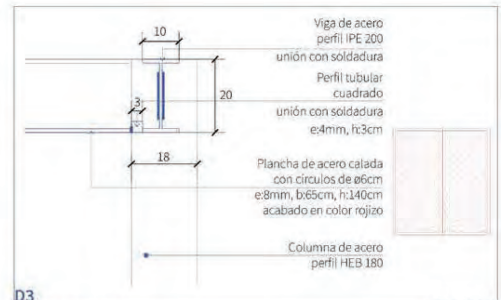
D3 Panel de techo
