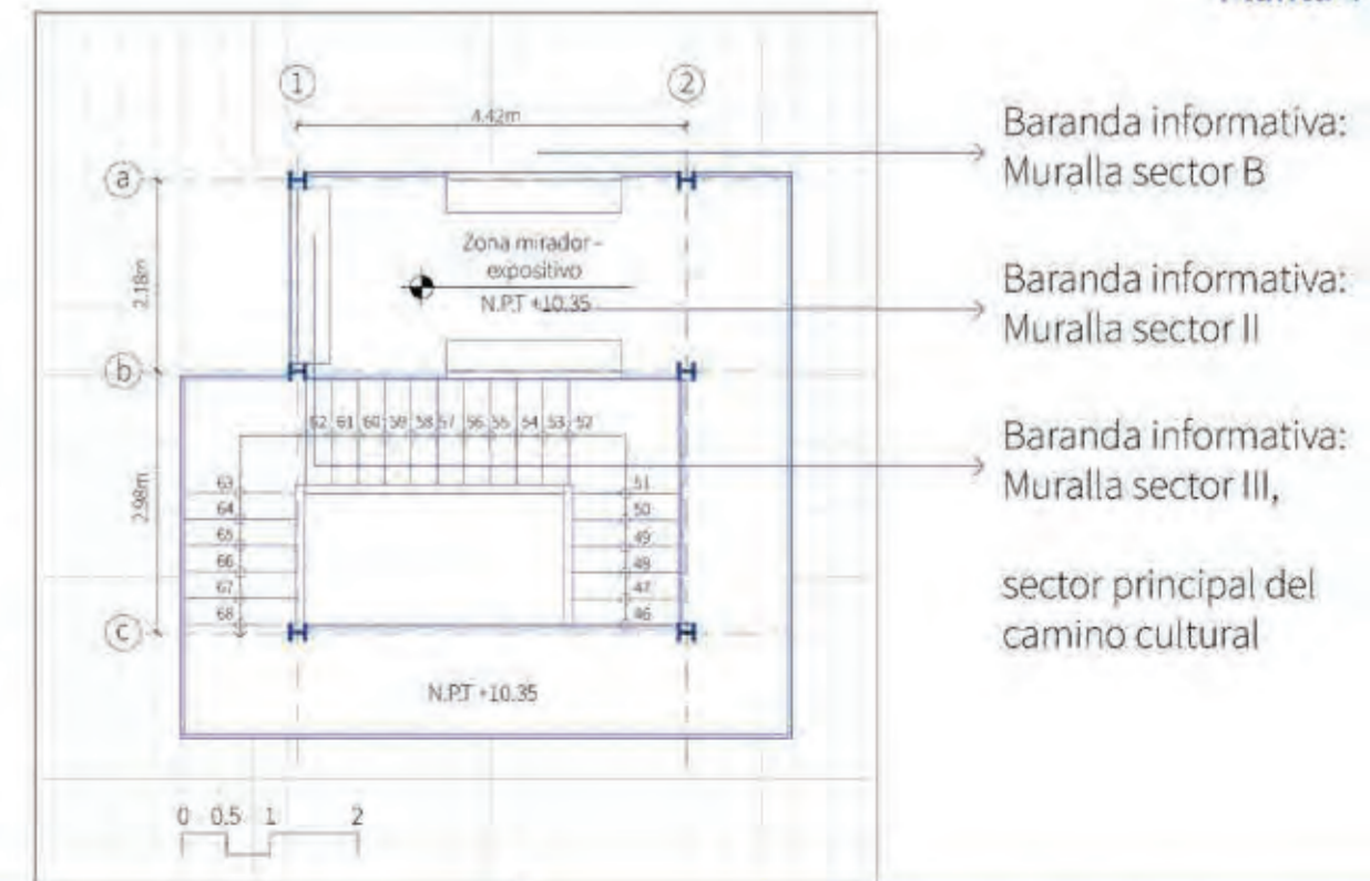
Planta 4
