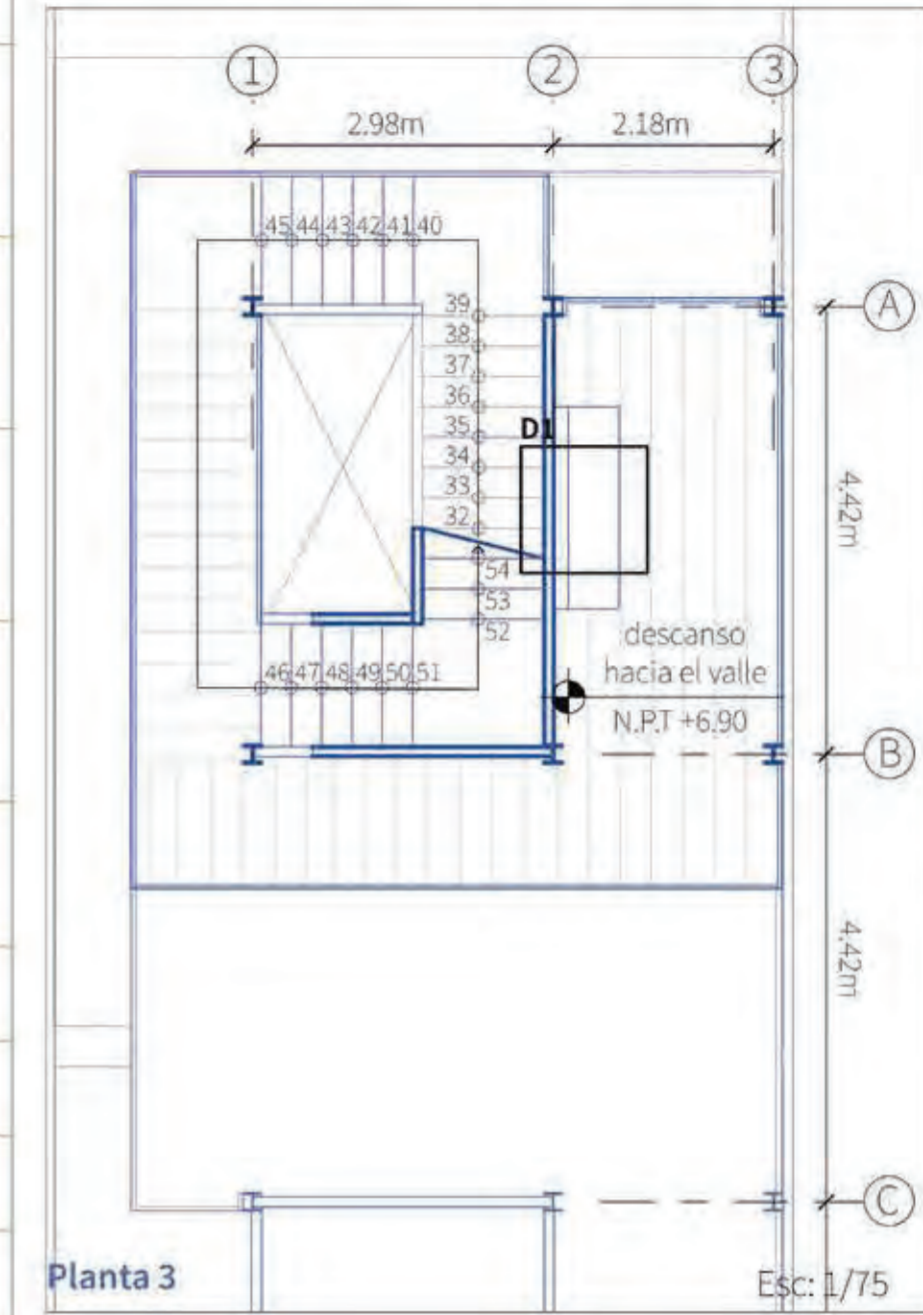
D1 baranda - asiento
