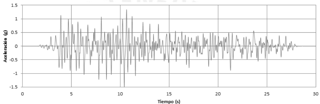
Figura 2. Aceleración en la mesa vibradora medida en ensayo con desplazamiento pico D = 130 mm
