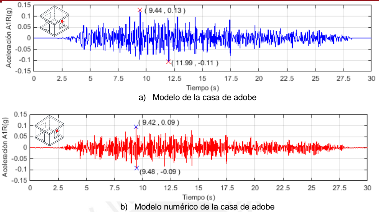
Figura 15. Respuesta de aceleraciones relativas a la base medida en la parte superior del muro derecho
