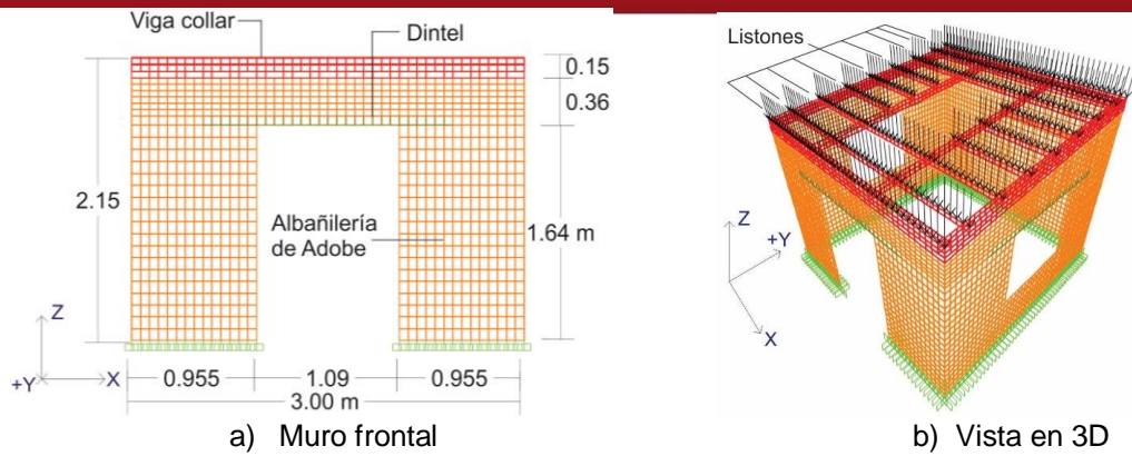
Figura 13. Modelo numérico representativo de la casa de adobe
