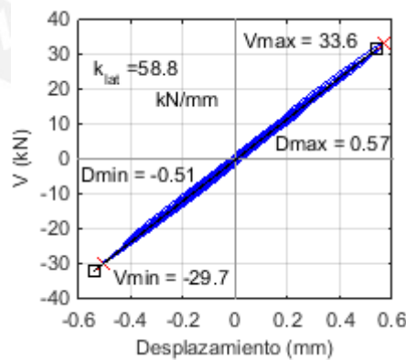
Figura 18. Cortante basal vs. desplazamiento promedio del modelo numérico al finalizar la primera fase de la simulación
