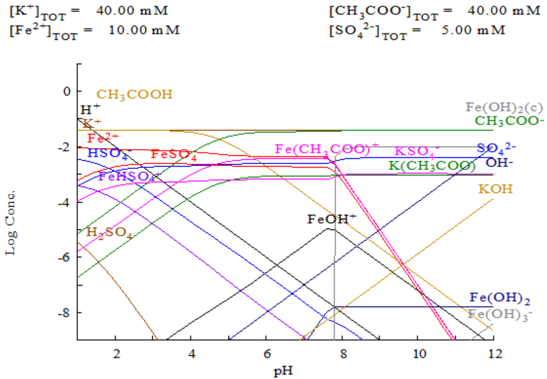
Figura XXVIII: Diagrama completo pH vs. log de concentración, construido con HydroMedusa, considerando todos los reactivos, con sus respectivas concentraciones, de la celda electroquímica de trabajo
