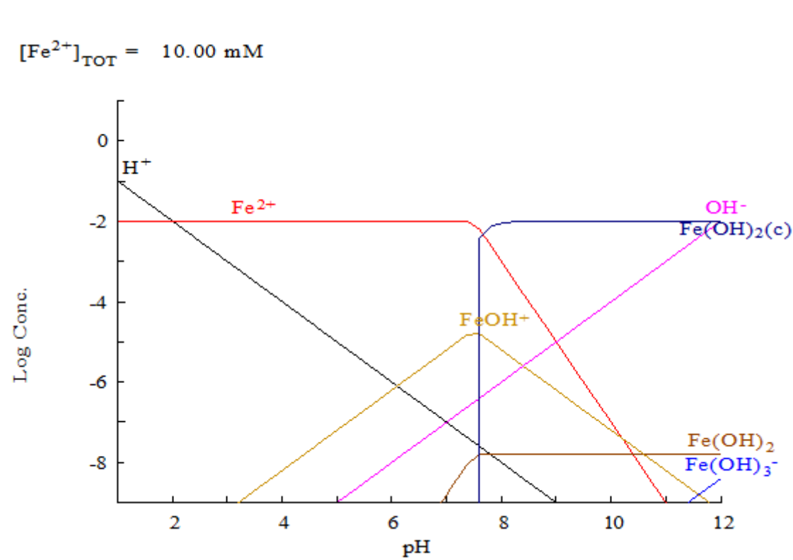
Figura XXVII: Diagrama completo pH vs. \log [Fe^{2+}] . Construido con el software HydroMedusa, considerando una concentración de Fe^{2+} total de 0,01M
