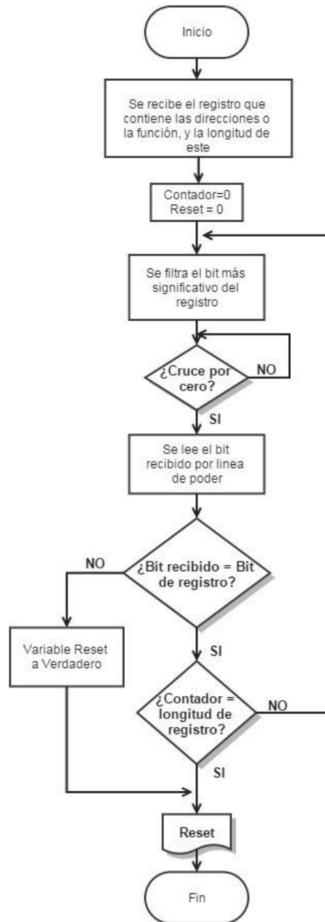
Figura 3. 29 Diagrama de Flujo de Recepción de Pulsos PLC
