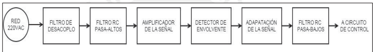
Figura 3. 11 Diagrama de Bloques del Circuito Detector de Pulsos PLC
