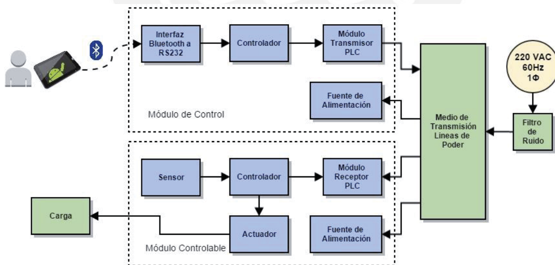
Figura 3. 1 Diagrama de bloques del Sistema Domótico
