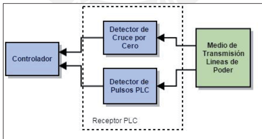
Figura 3. 10 Diagrama de Bloques del Receptor de Comunicación por Línea de Poder
