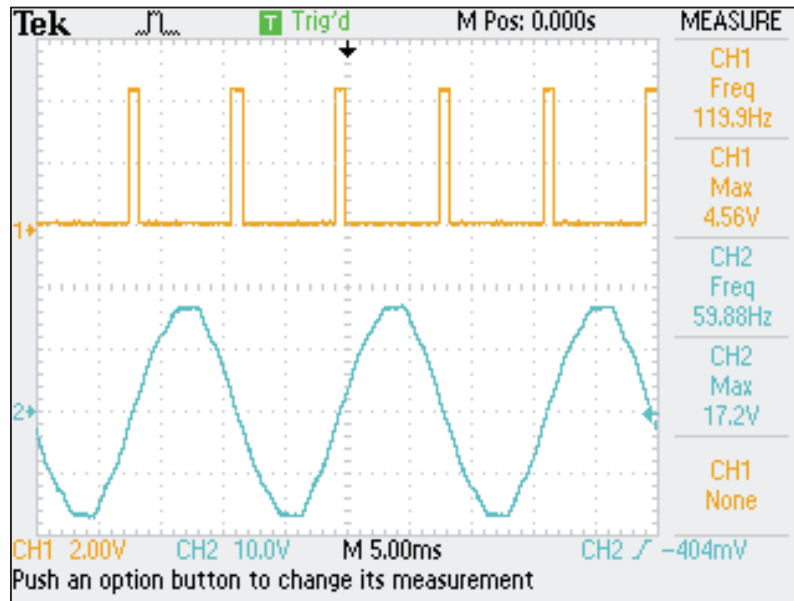
Figura 4. 1 Prueba del Circuito Detector de Cruce por Cero
