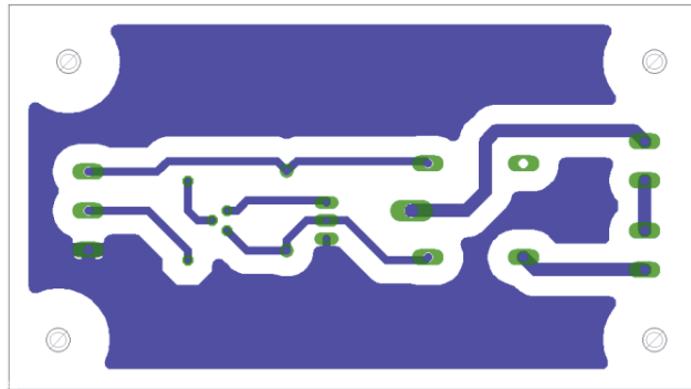
Figura 3. 17 Capa de Cobre Posterior del Circuito de Control de Tomacorrientes
