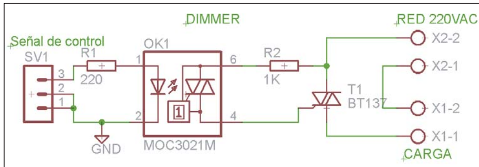
Figura 3. 13 Esquemático del Circuito de Control de Iluminación
