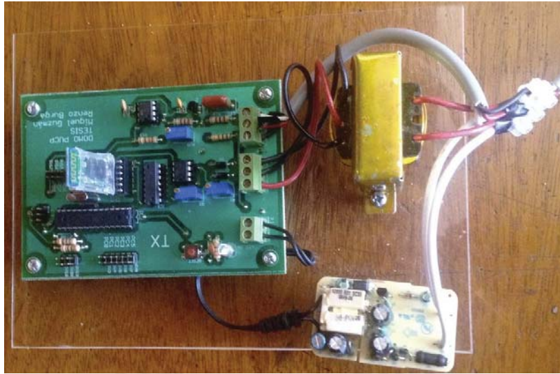
Figura 4. 16 Módulo de Control
