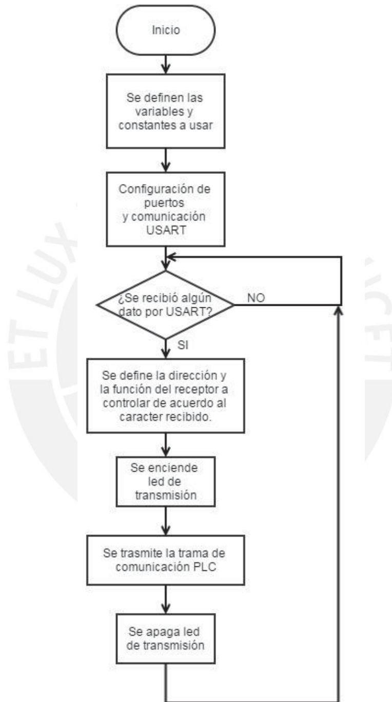
Figura 3. 26 Diagrama de Flujo del Programa Principal del Módulo de Control
