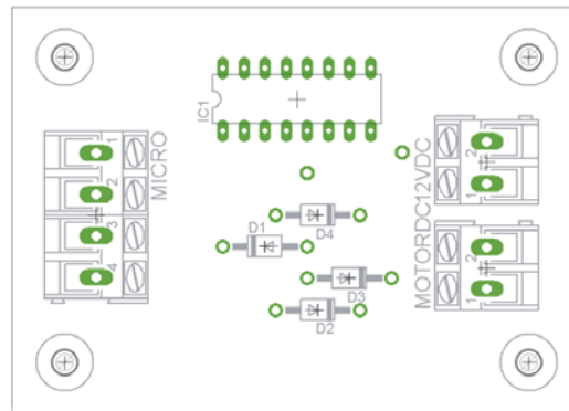
Figura 3. 21 Capa de Componentes Superior del Circuito de Control de Cortinas
