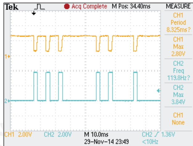
Figura 4. 5 Prueba Tras el Detector de Envoltente del Circuito Detector de Pulsos PLC
