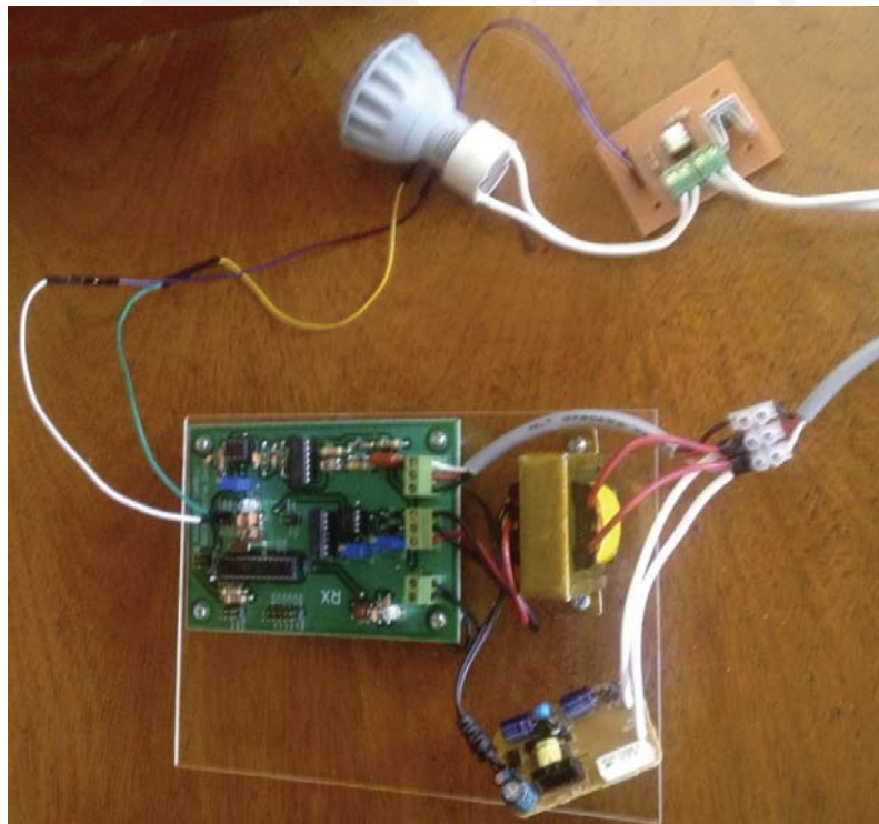
Figura 4. 17 Modulo Controlable - Control de Iluminación
