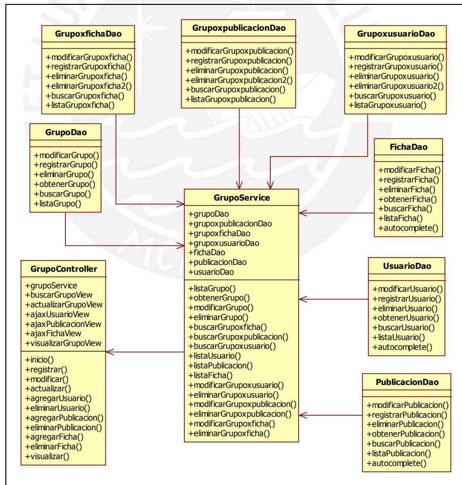
Imagen 3: Diagrama de Clase de Diseño del Módulo del Compartidos
