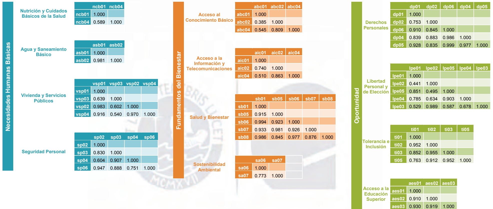
Figura 14. Correlación de los indicadores del IPS del Distrito de Huarmey 2019. Adaptado de Encuesta IPS Huarmey 2019.
