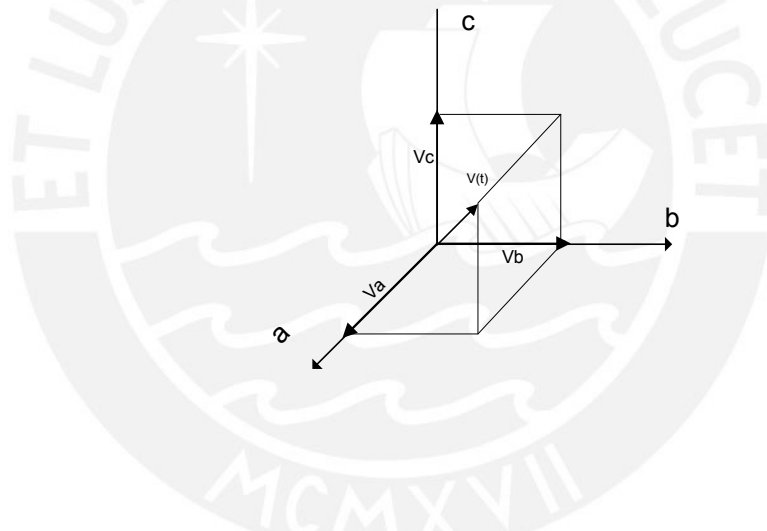
Figura 2. Representación de vector espacial mediante ejes ortogonales a, b y c.
